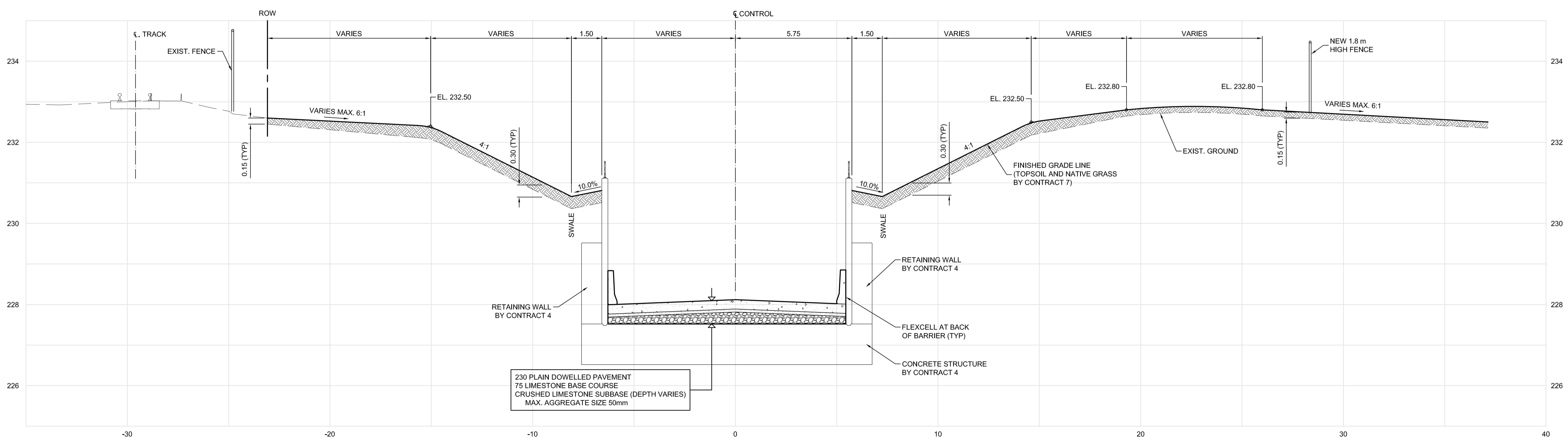
B SECTION - STA. 11+740 SCALE: H = 1:100 V = 1:50
