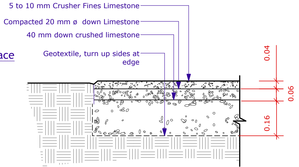
3 Crusher Fines Paving L-7 Scale: 1:10
