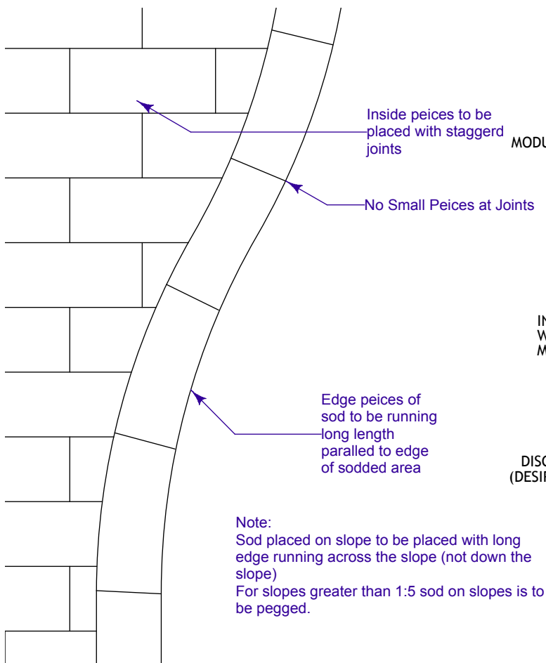
5 Sod Pattern L-7 Scale: 1:50
