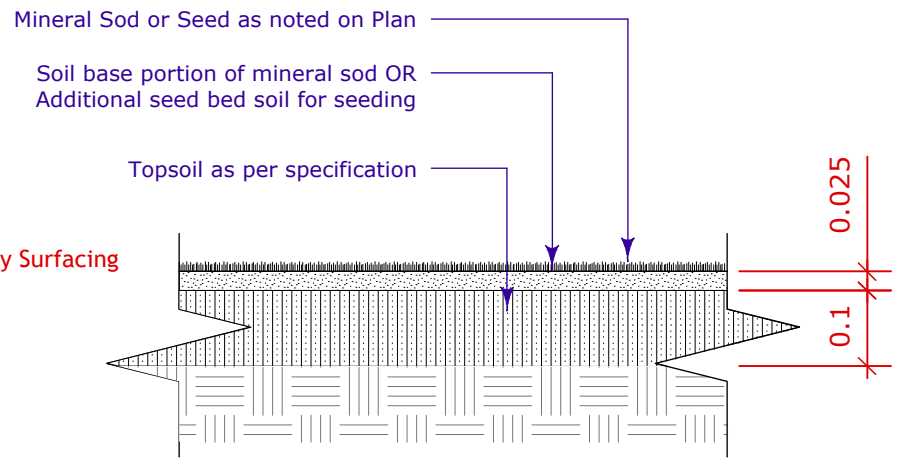
4 Sod Detail L-7 Scale: 1:10
