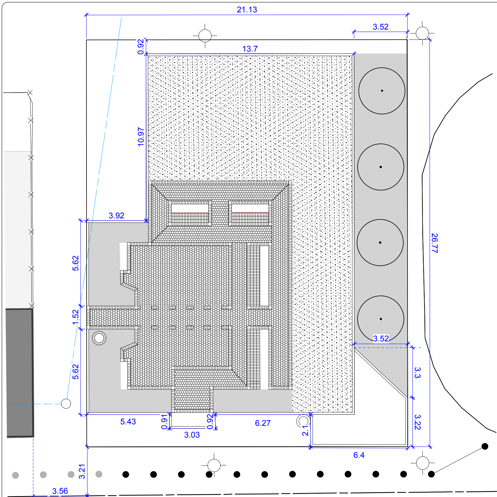
SITE LAYOUT Scale - 1:150
