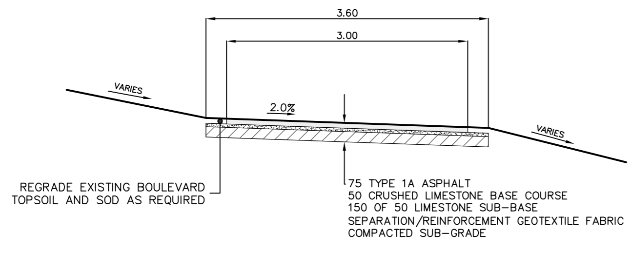
SECTION A-A SCALE N.T.S.
