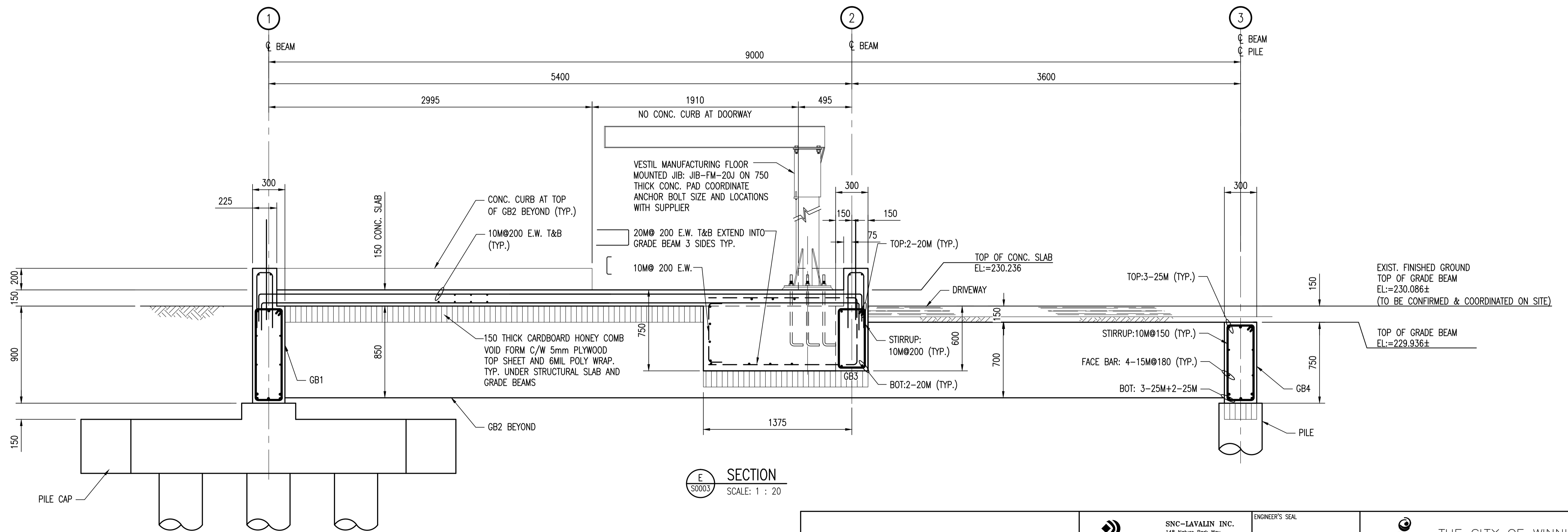
D SECTION SCALE: 1 : 20
