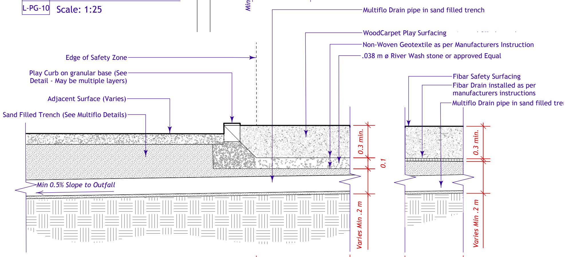
2 Section B L-PG-10 Scale: 1:20
