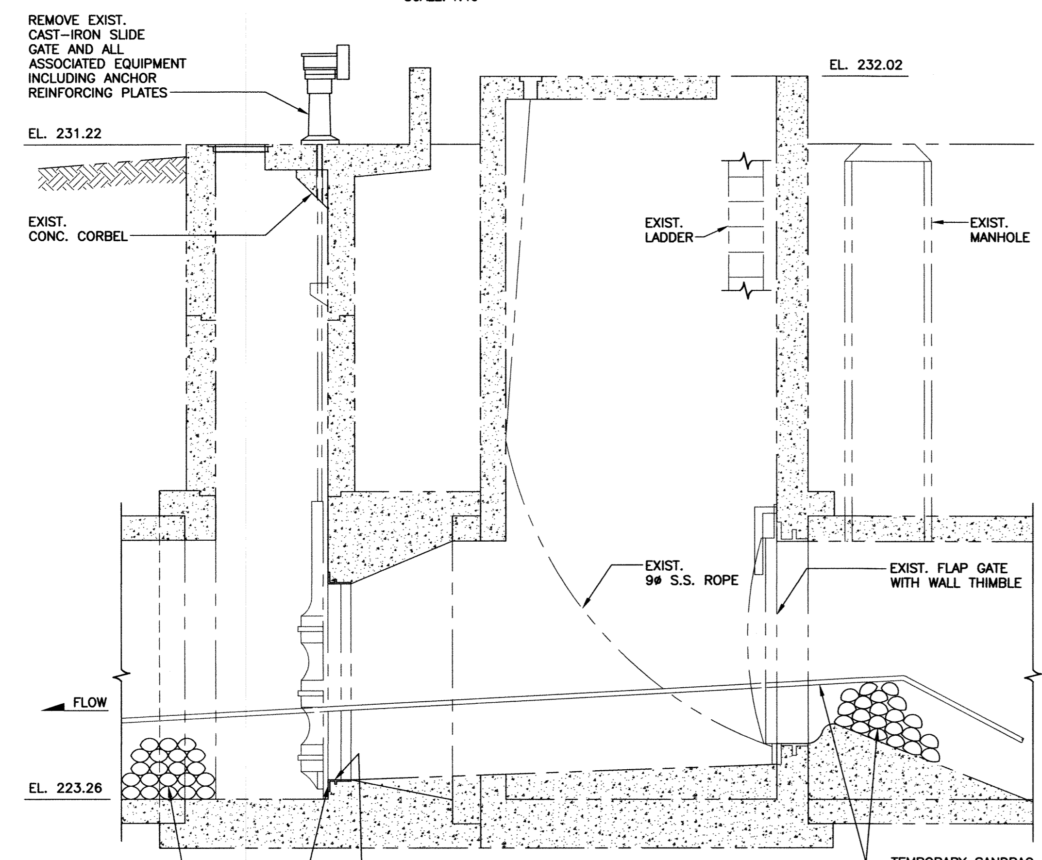
SECTION A-A SCALE: 1:40
