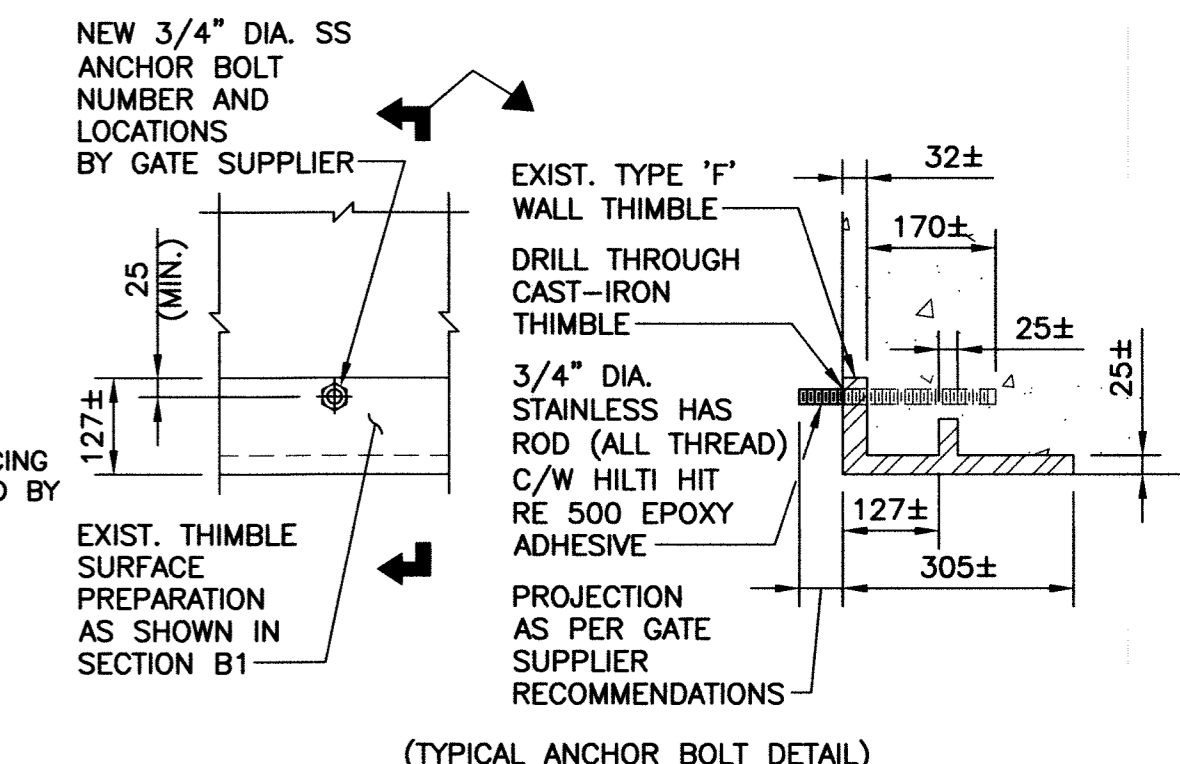
C DETAIL SCALE: 1:10
