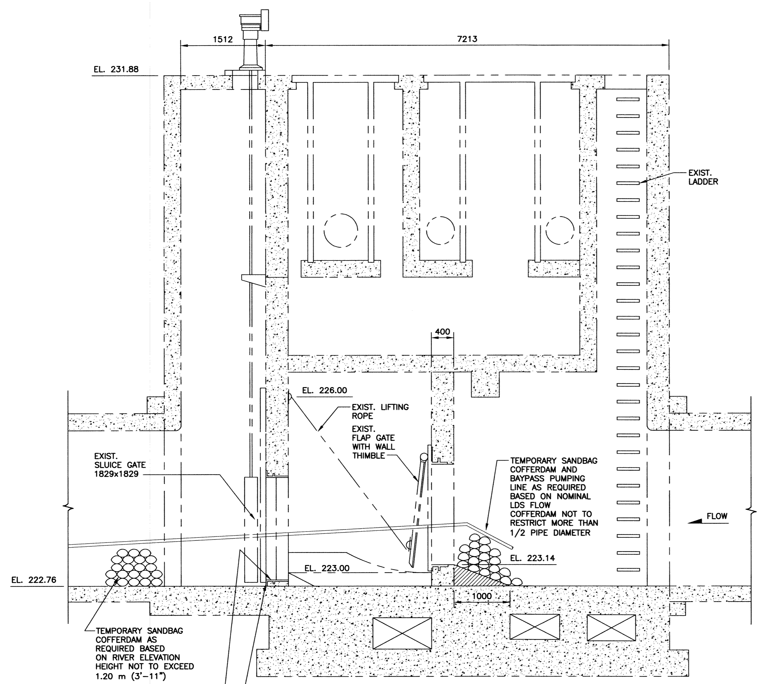
A SECTION SCALE: 1:40
