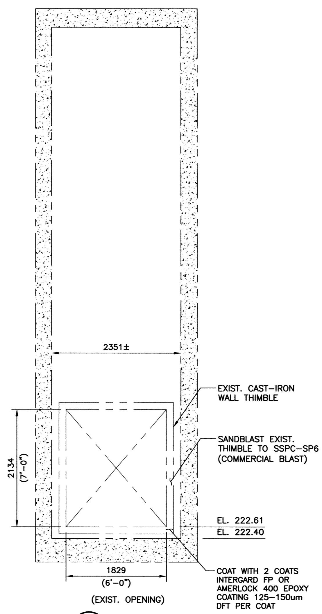
SECTION B1 SCALE: 1:40
