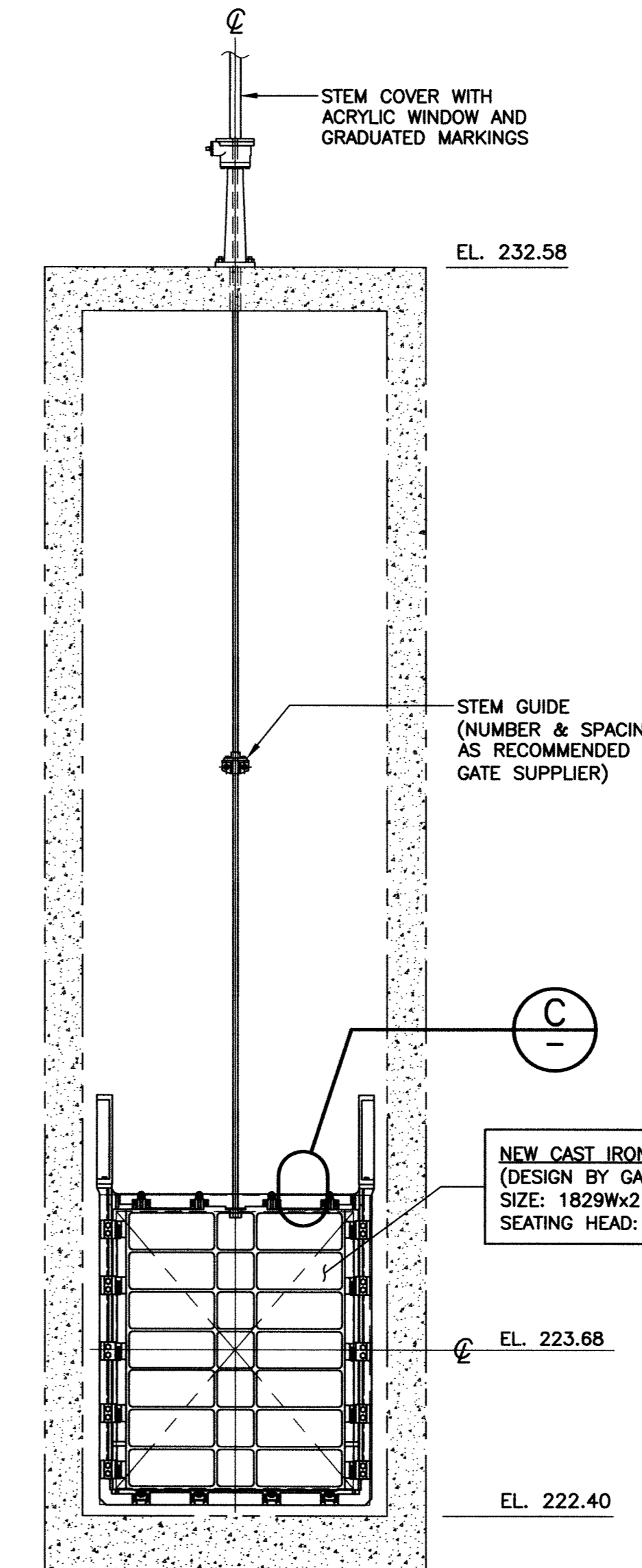
SECTION B2 SCALE: 1:40
