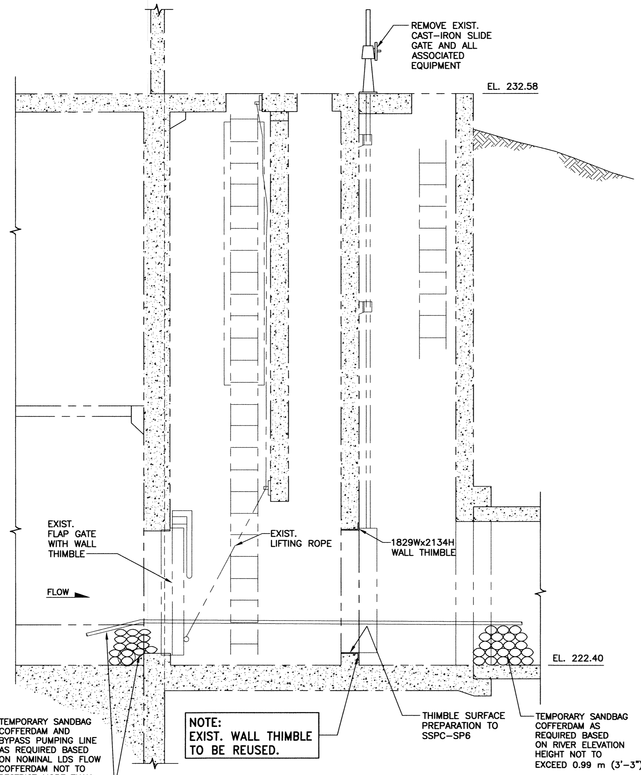
SECTION A SCALE: 1:40
