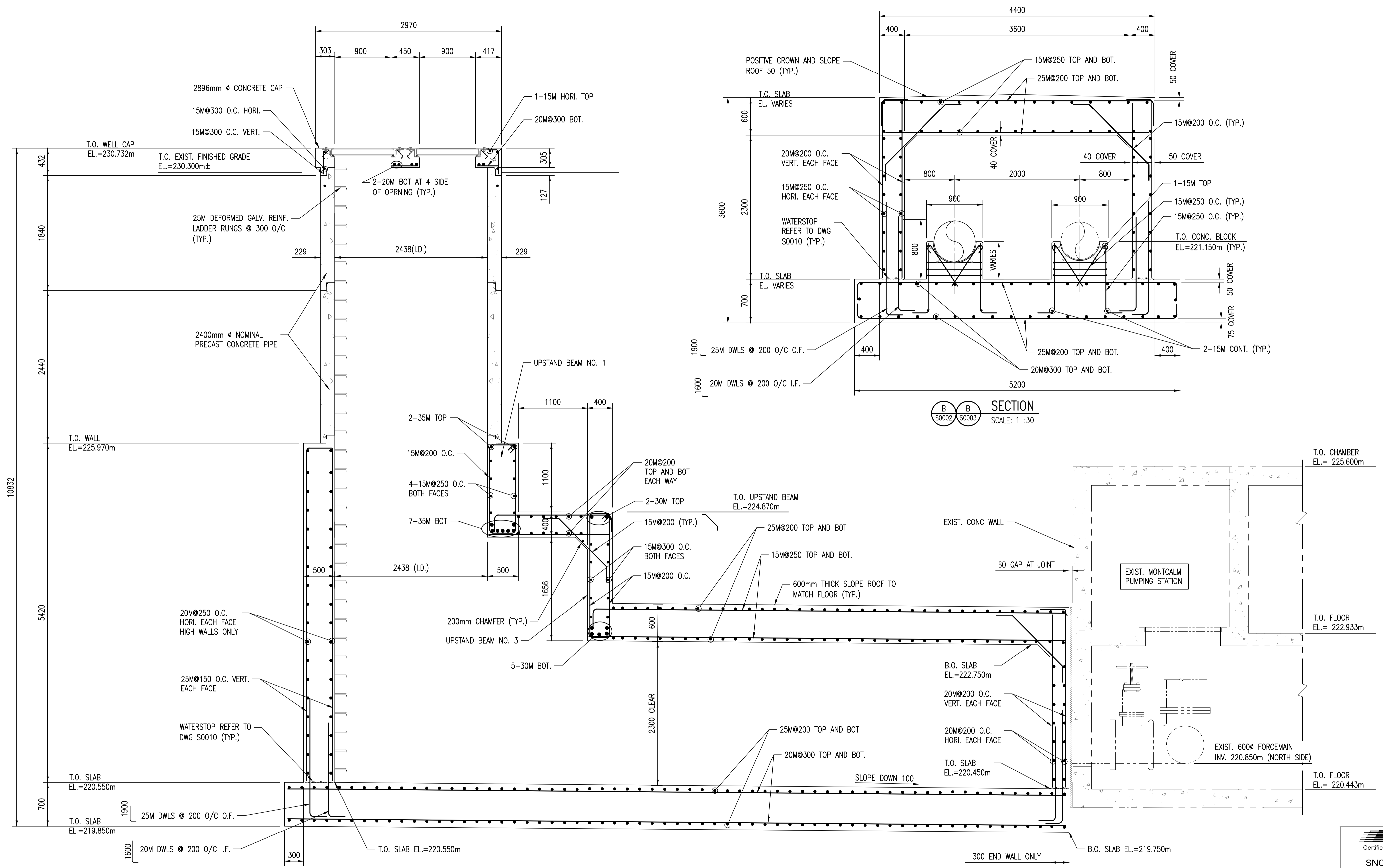
SECTION A-A SCALE: 1 : 30
