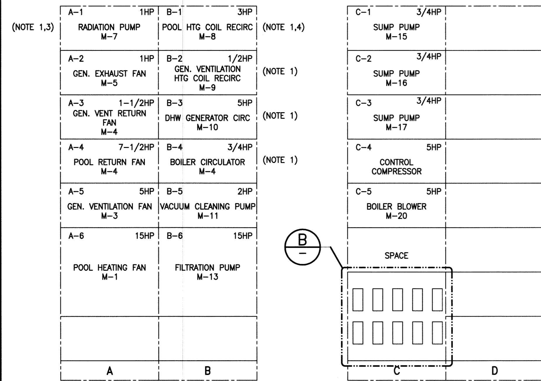
A MCC-1 ELEVATIONS SCALE: N.T.S.
