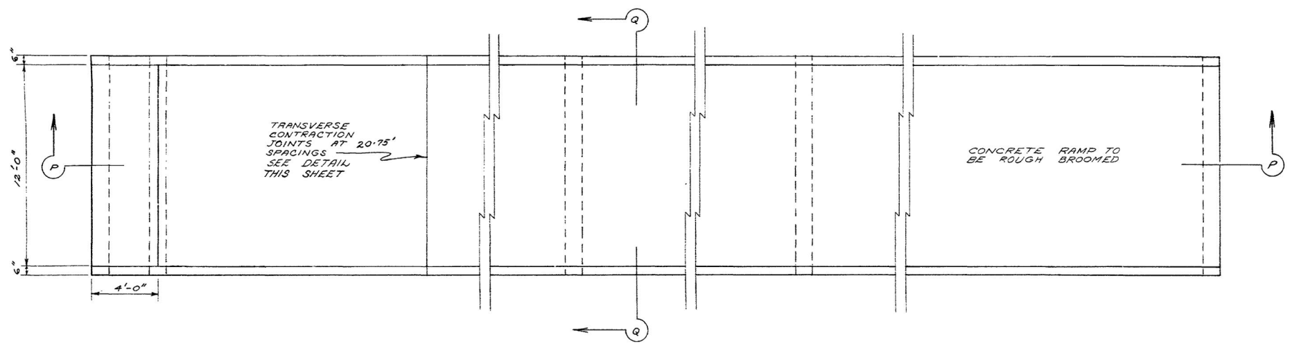
PLAN SCALE: 1/4" = 1'-0"
