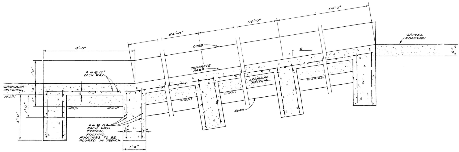
SECTION "P-P" SCALE: 1" = 1'-0"
