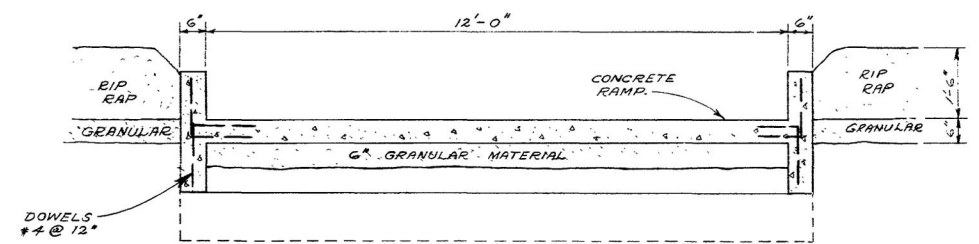
SECTION "Q-Q" SCALE: 1/2" = 1'-0"
