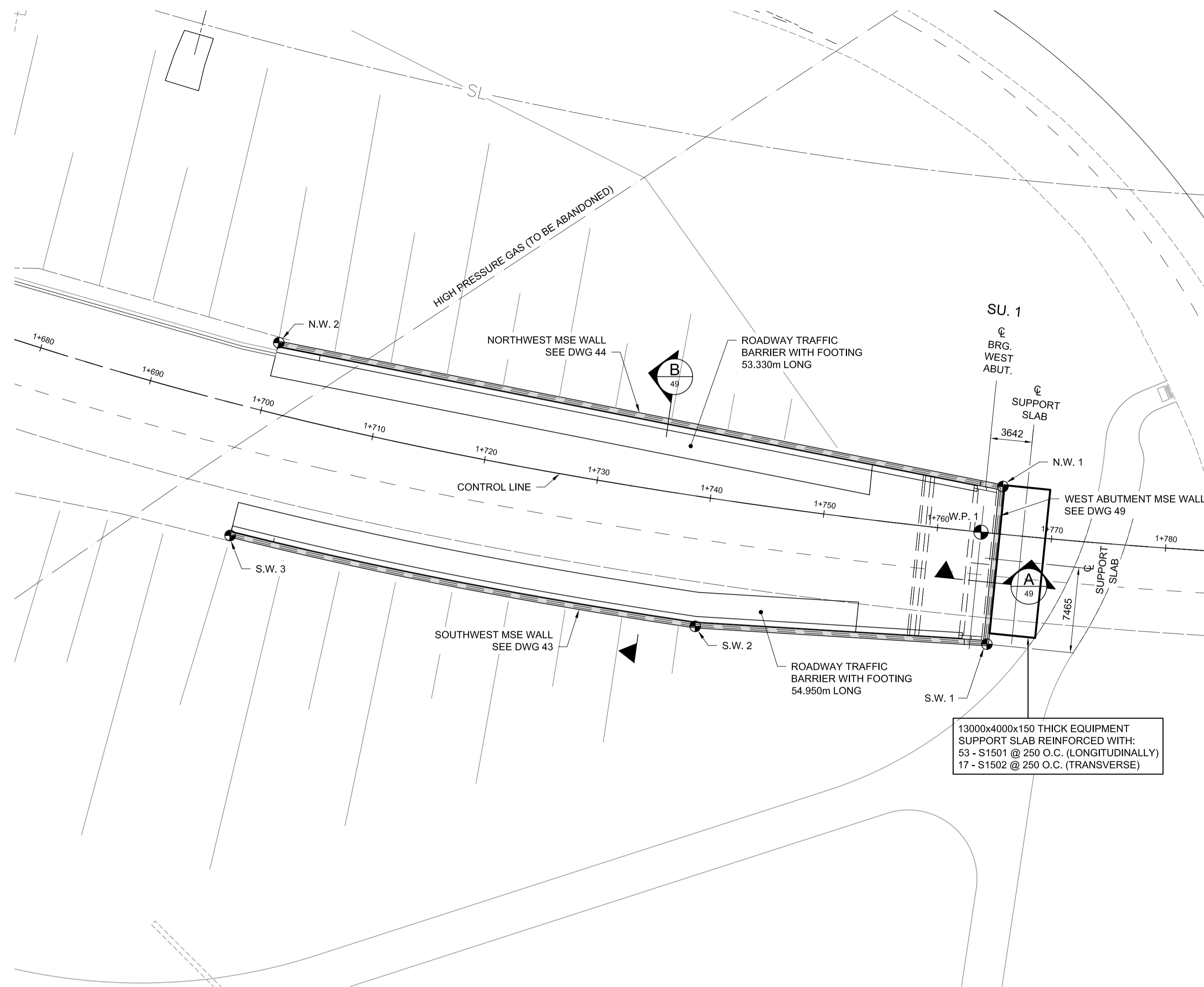
PLAN 1:250
