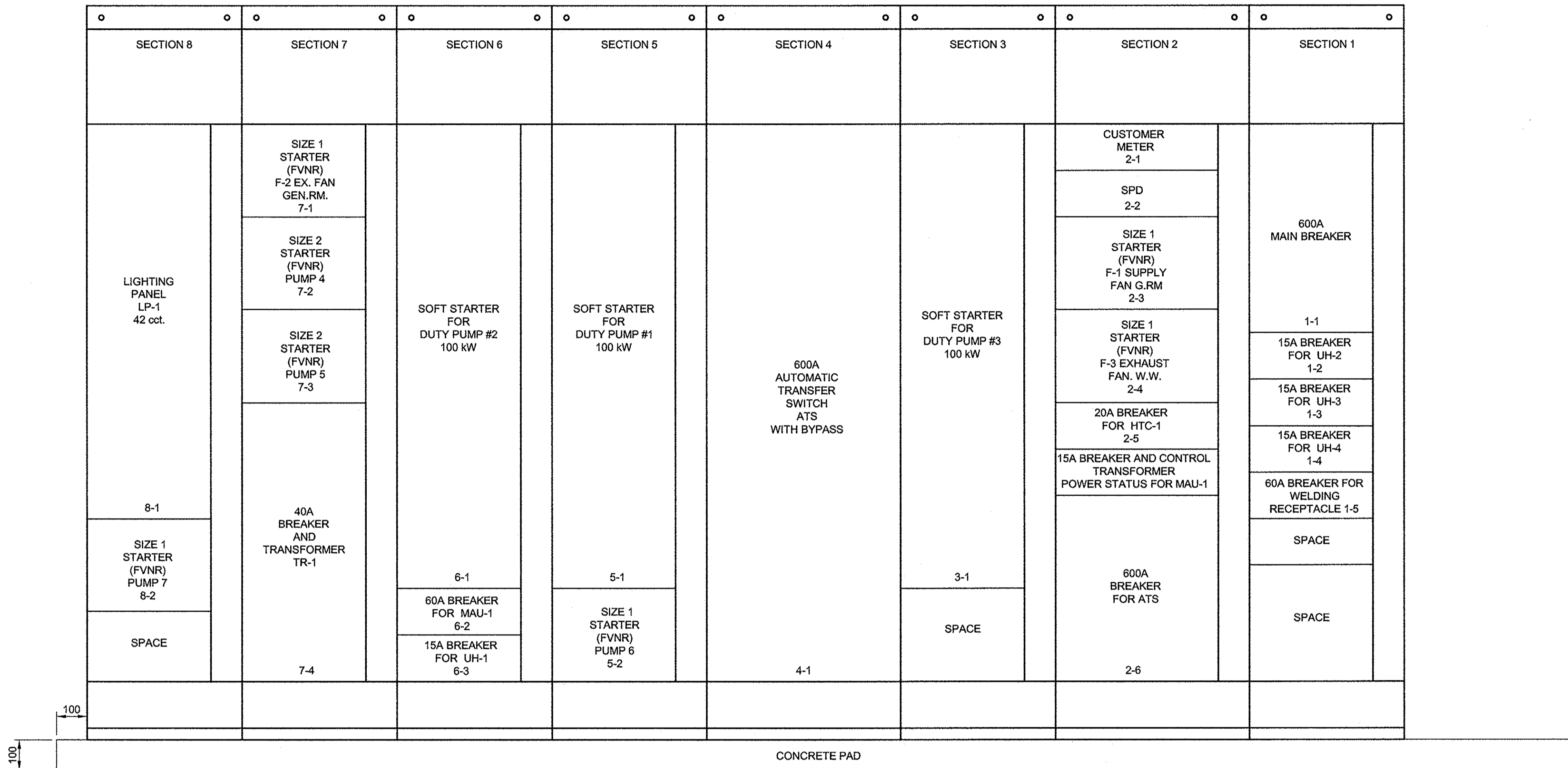
MCC ELEVATION Scale N.T.S
