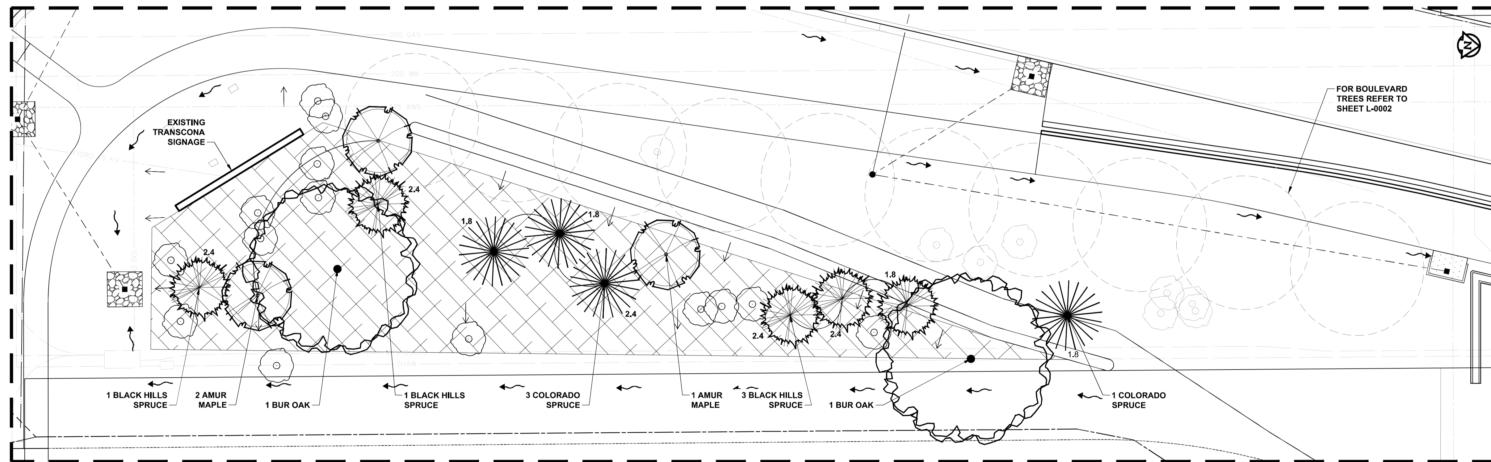
2 ENLARGEMENT L-0002 Scale 1:200
