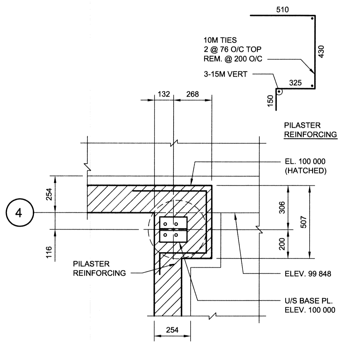
6 DETAIL - PL7 1:15
