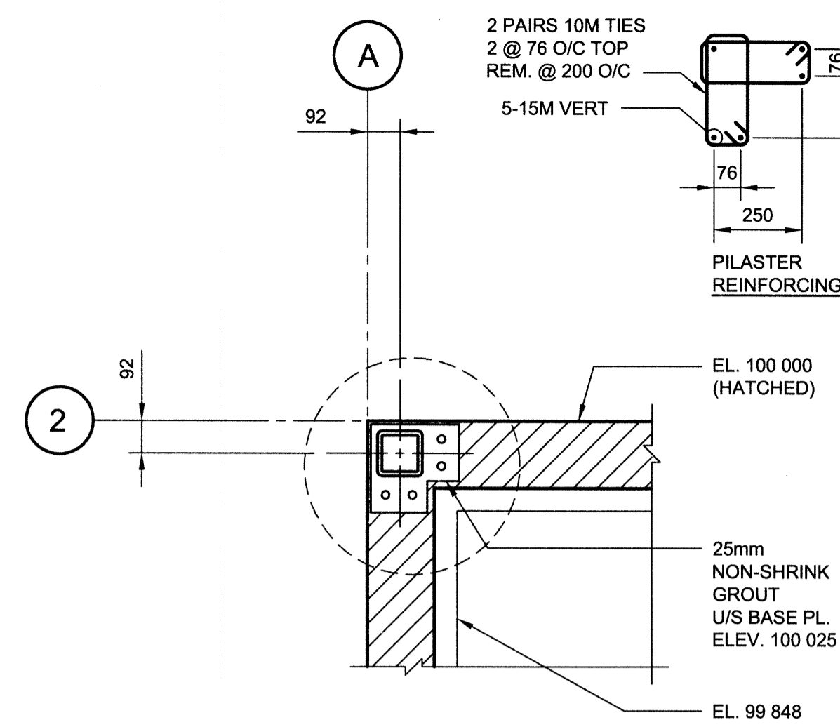
1 DETAIL - PL1 1:15
