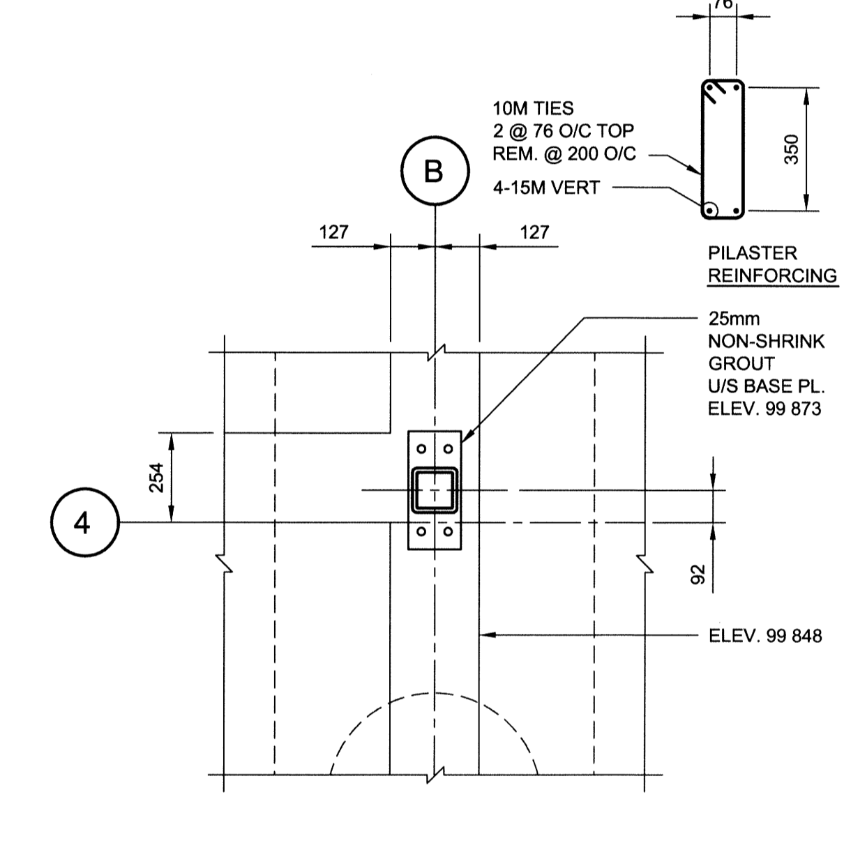
7 DETAIL - PL8 1:15
