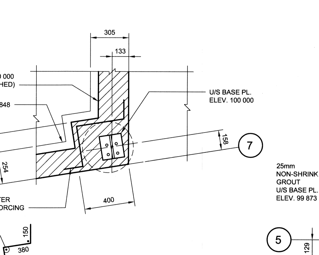
13 DETAIL - PL13 1:15
