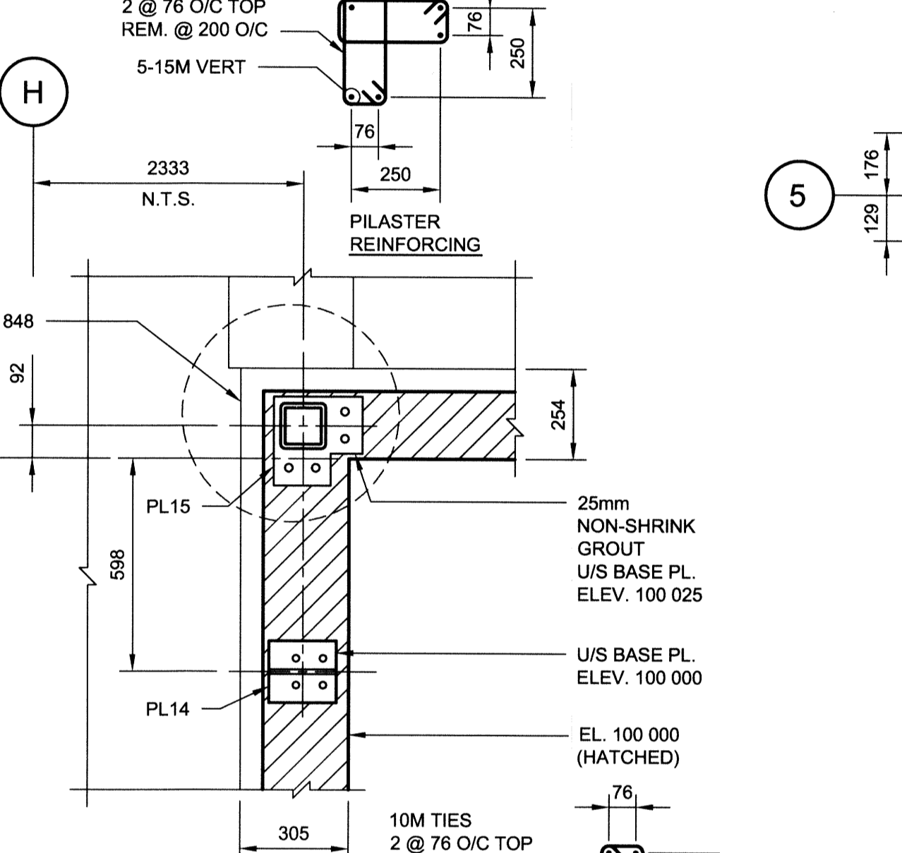
9 DETAIL - PL14 & PL15 1:15
