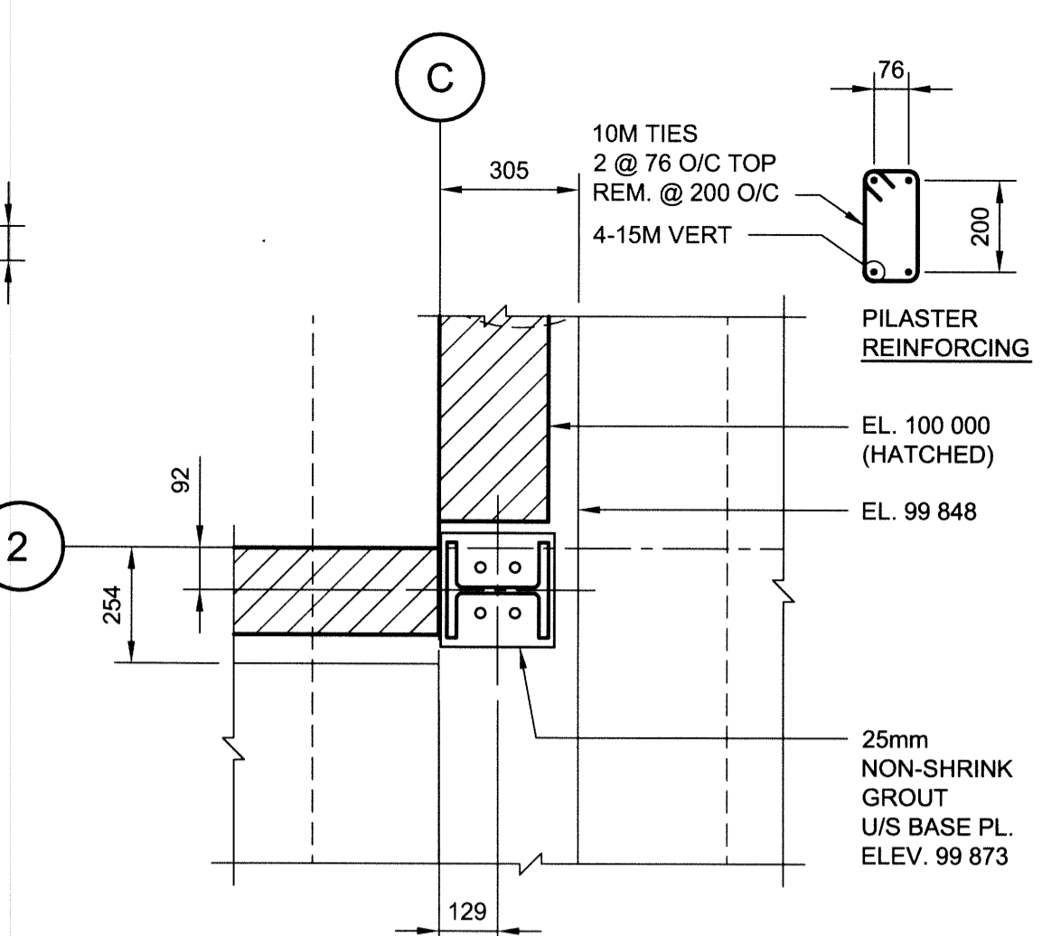
3 DETAIL - PL4 1:15
