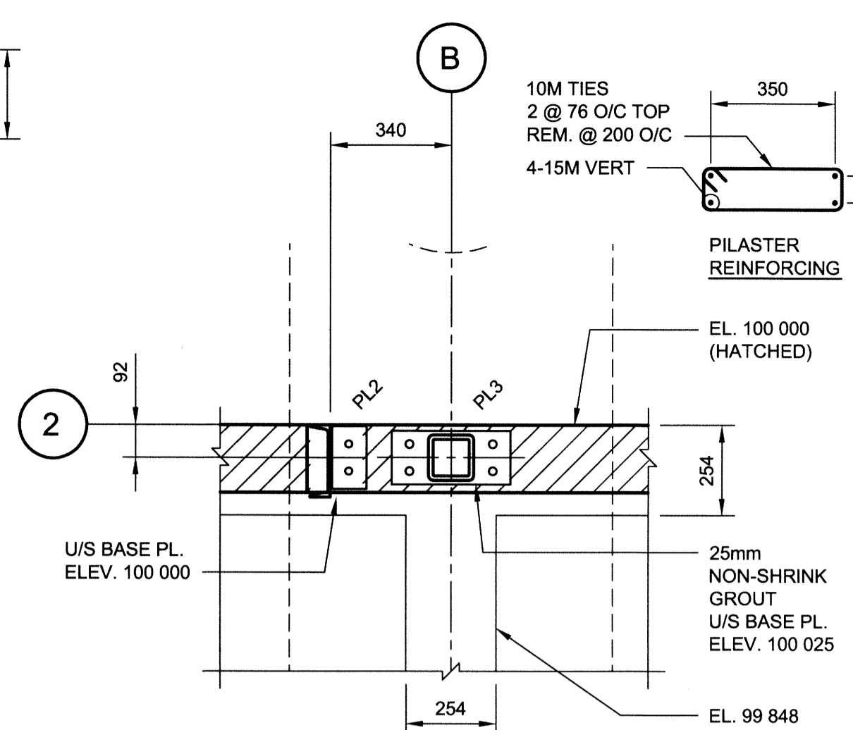
2 DETAIL - PL2 & PL3 1:15
