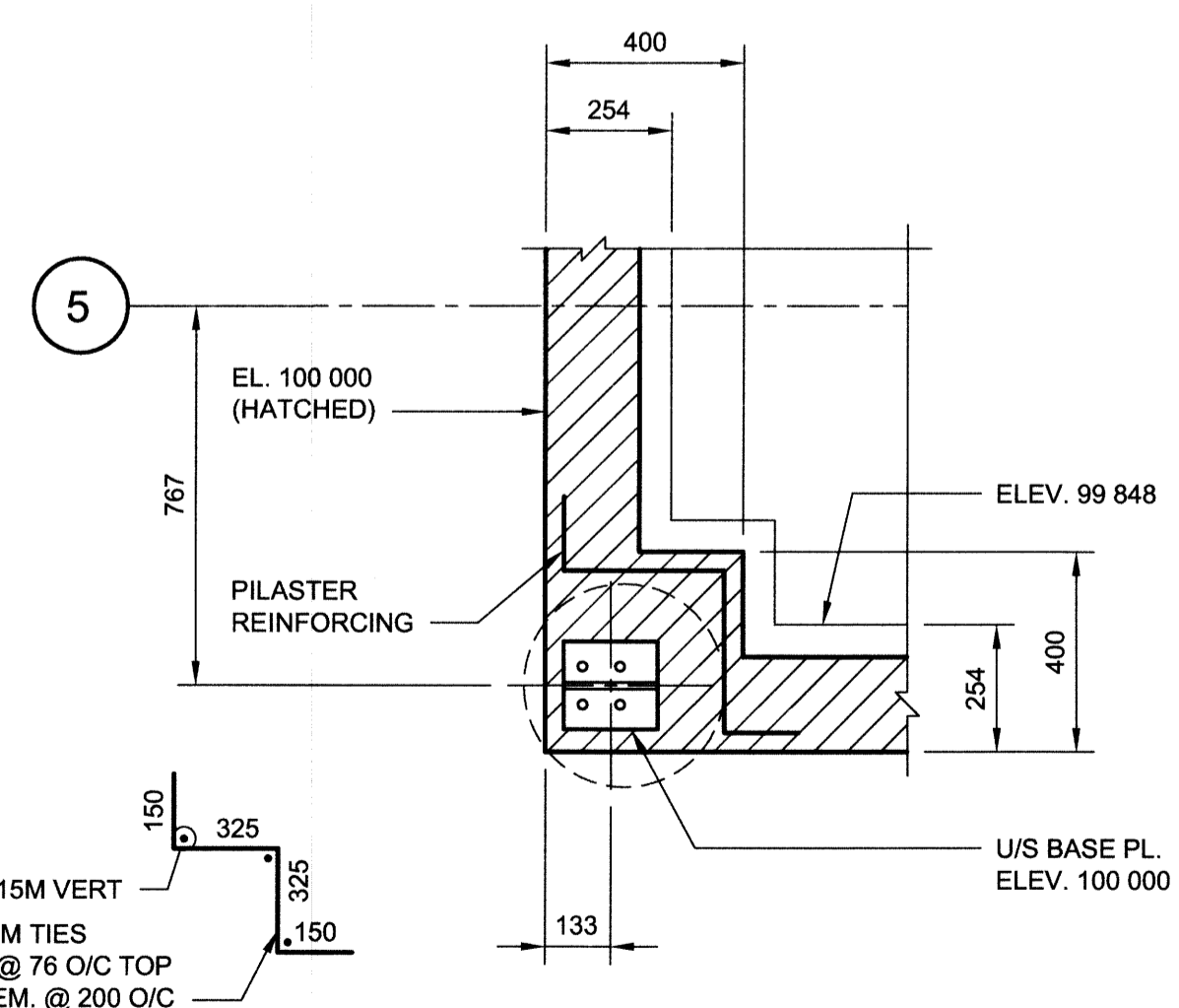
10 DETAIL - PL9 1:15
