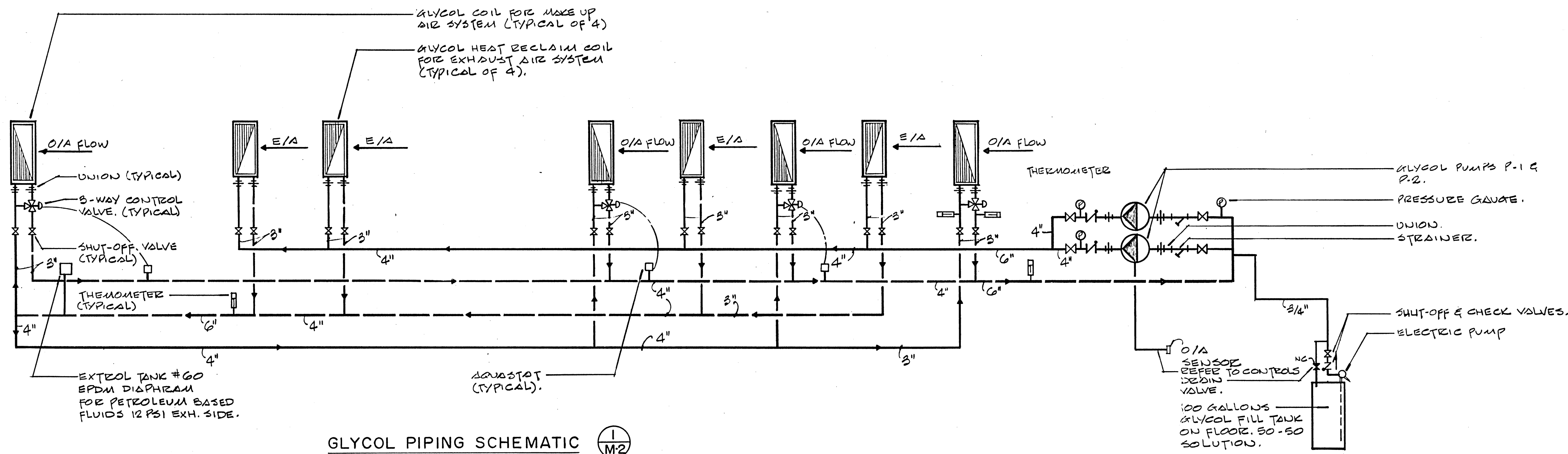
GLYCOL PIPING SCHEMATIC 1/M2 N.T.S.
