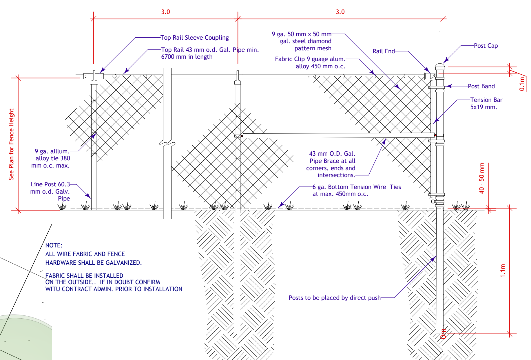
2 Chain Link Fence L-3 Scale: 1:20
