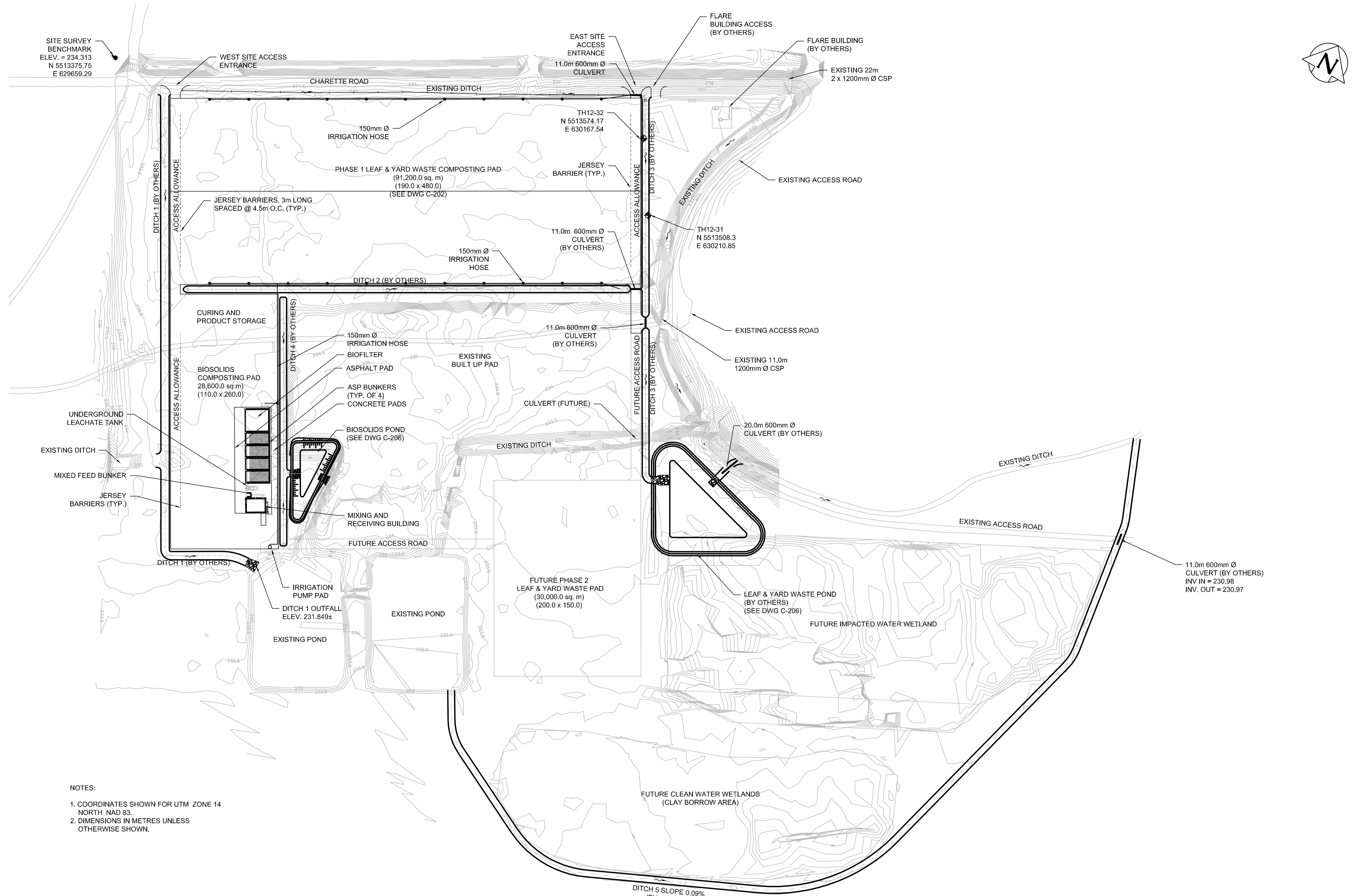
1 SITE PLAN 1:2000
