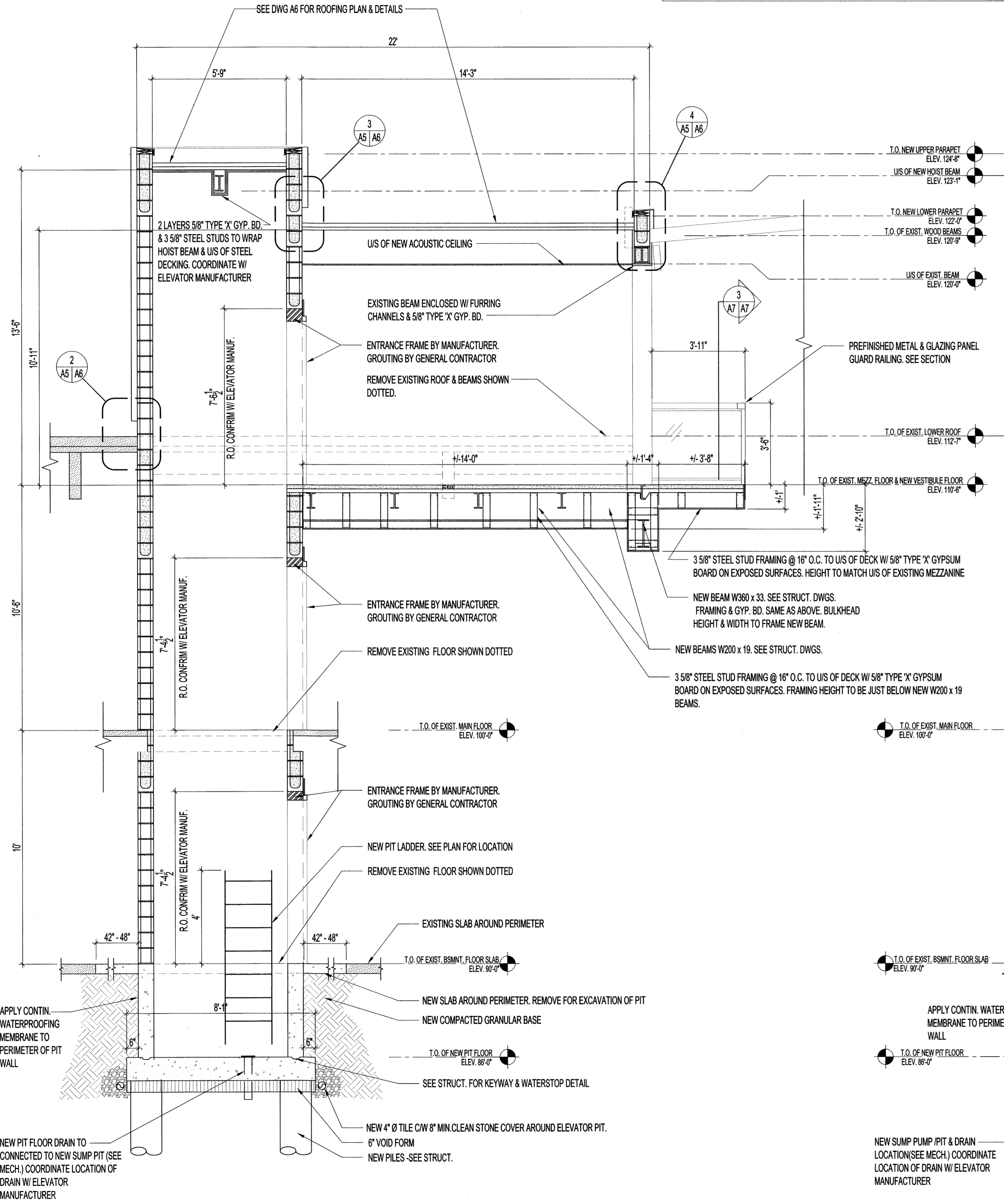
1 ELEVATOR SHAFT SECTION A2 | A5 / SCALE 3/8" = 1'-0"
