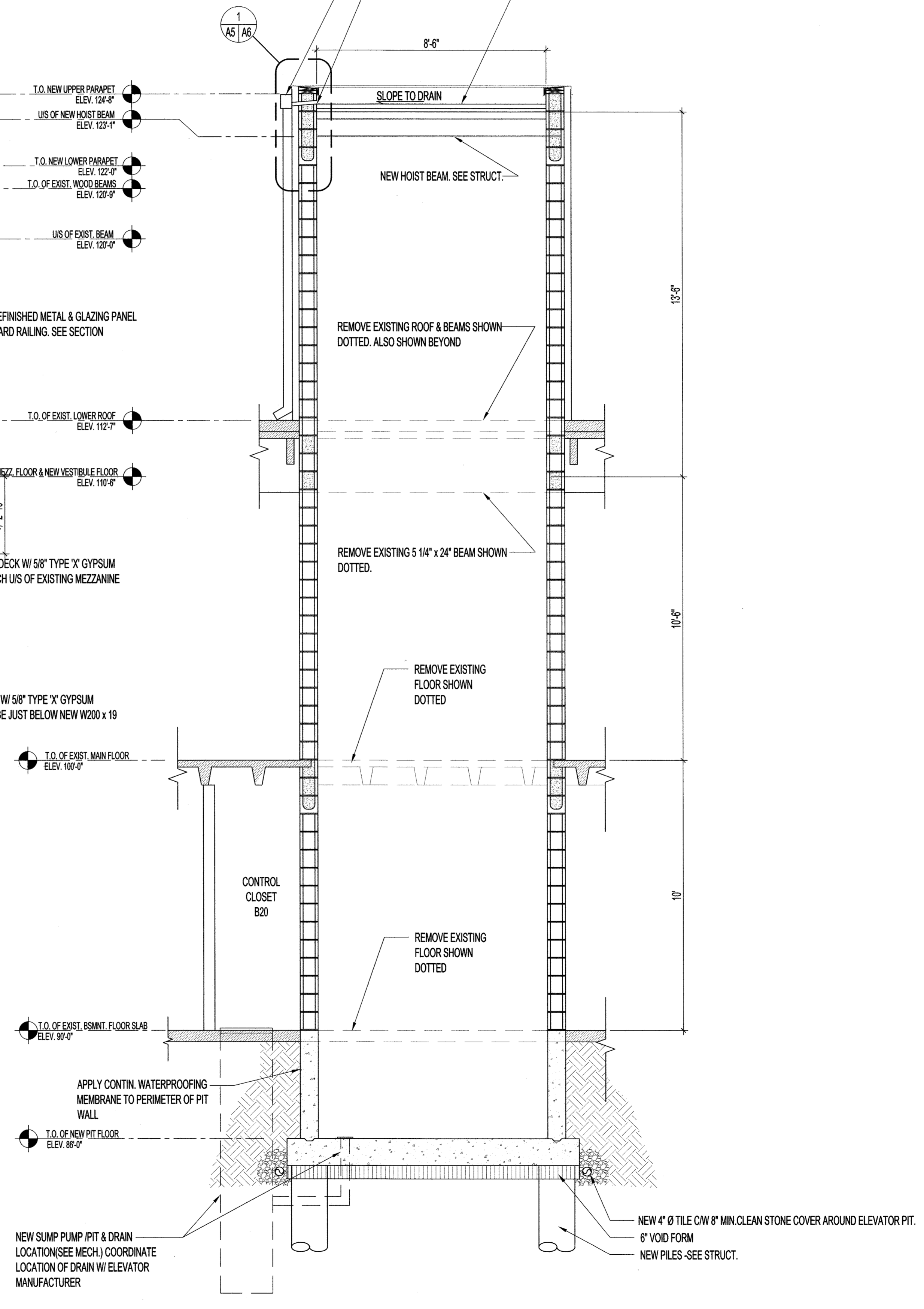
2 ELEVATOR SHAFT SECTION A2 | A5 / SCALE 3/8" = 1'-0"
