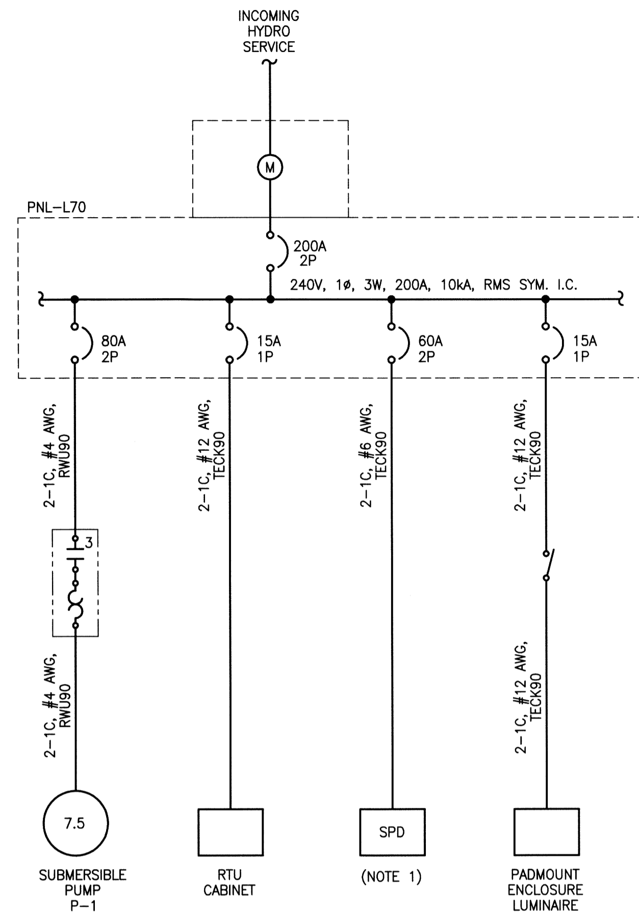
1 SINGLE LINE DIAGRAM SCALE: N.T.S.
