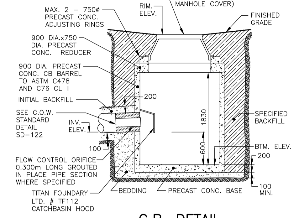
C.B. DETAIL N.T.S.
