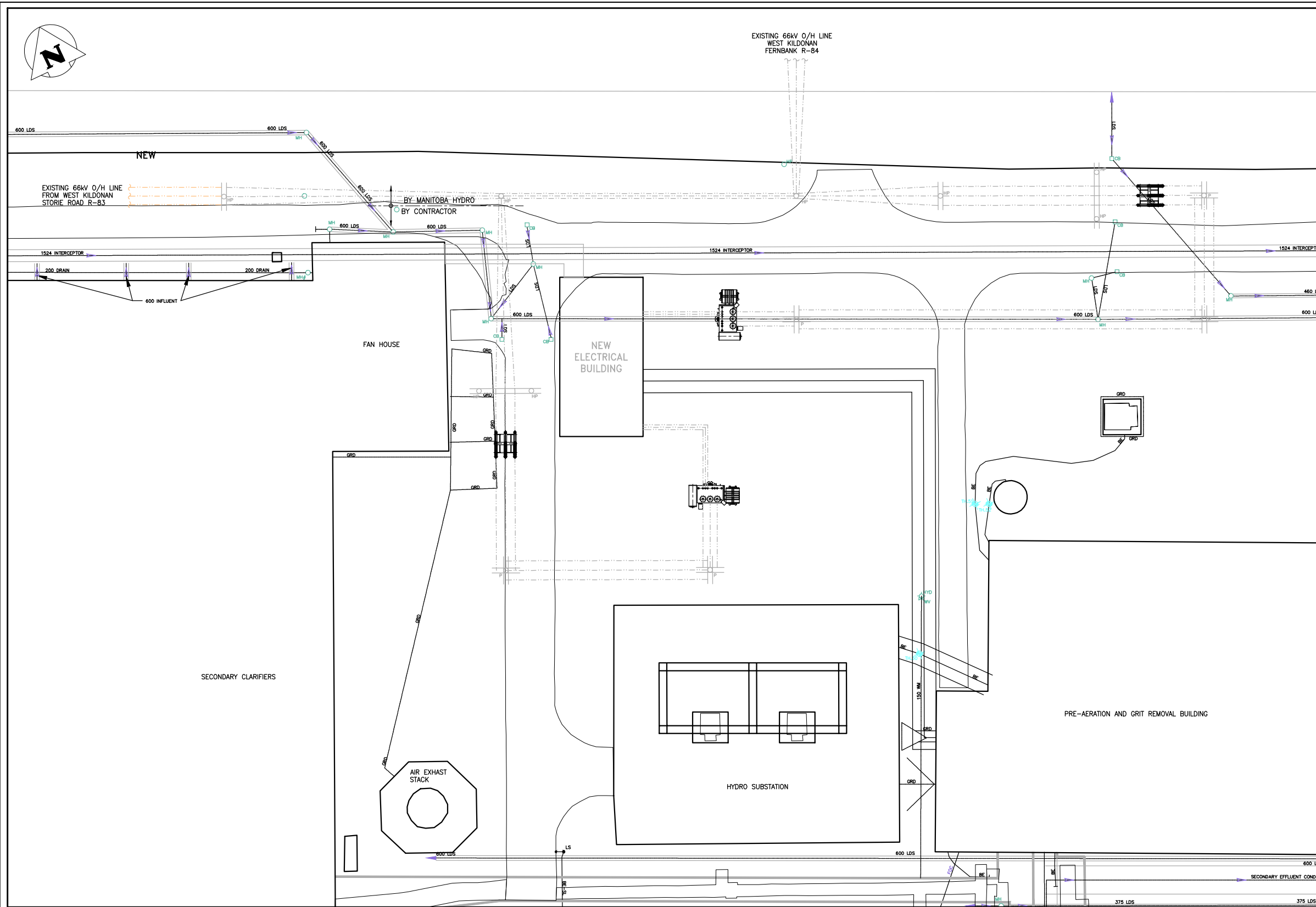
PLAN - COMPLETED WORK SCALE: N.T.S.
