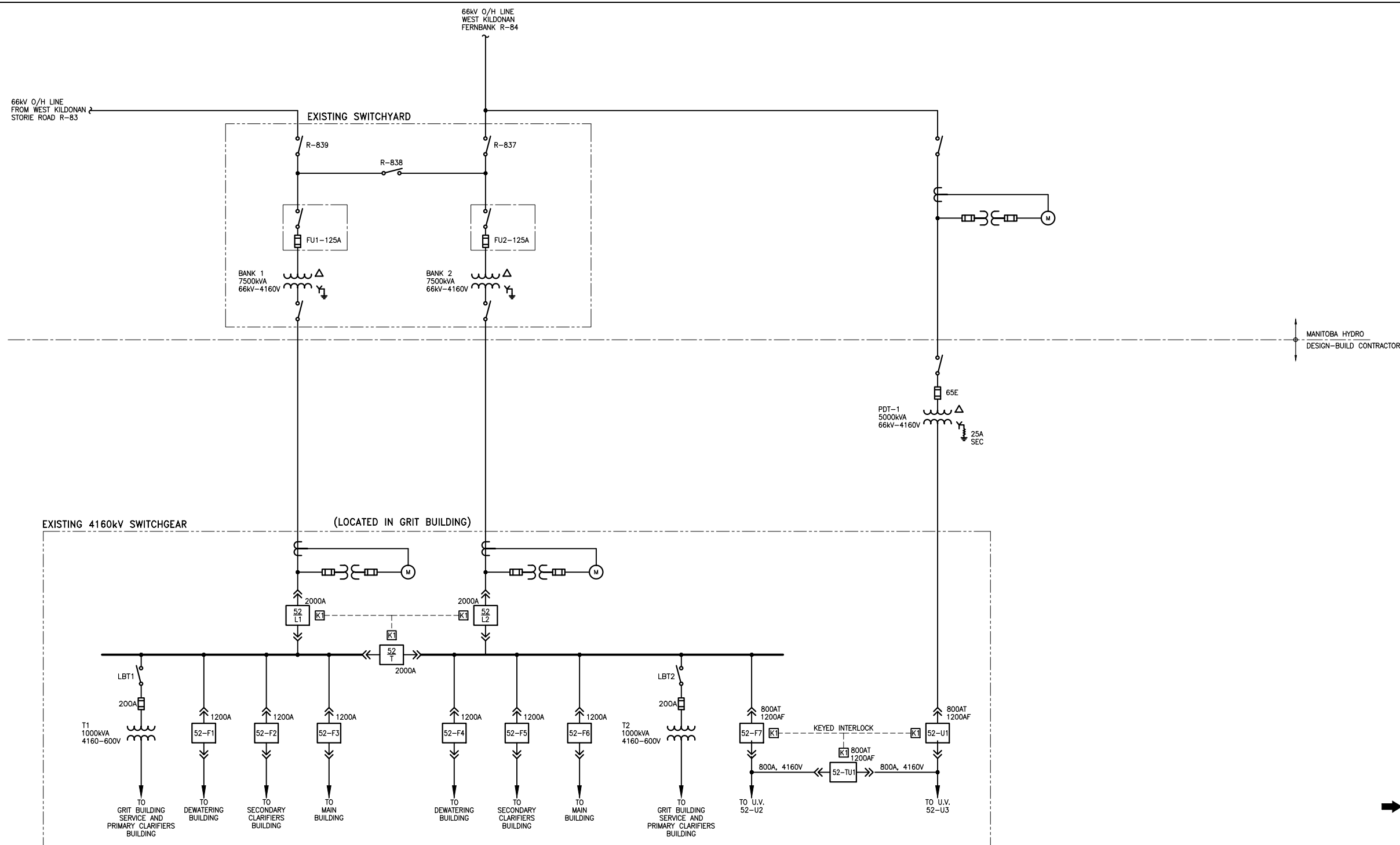
A SINGLE LINE DIAGRAM SCALE: N.T.S.
