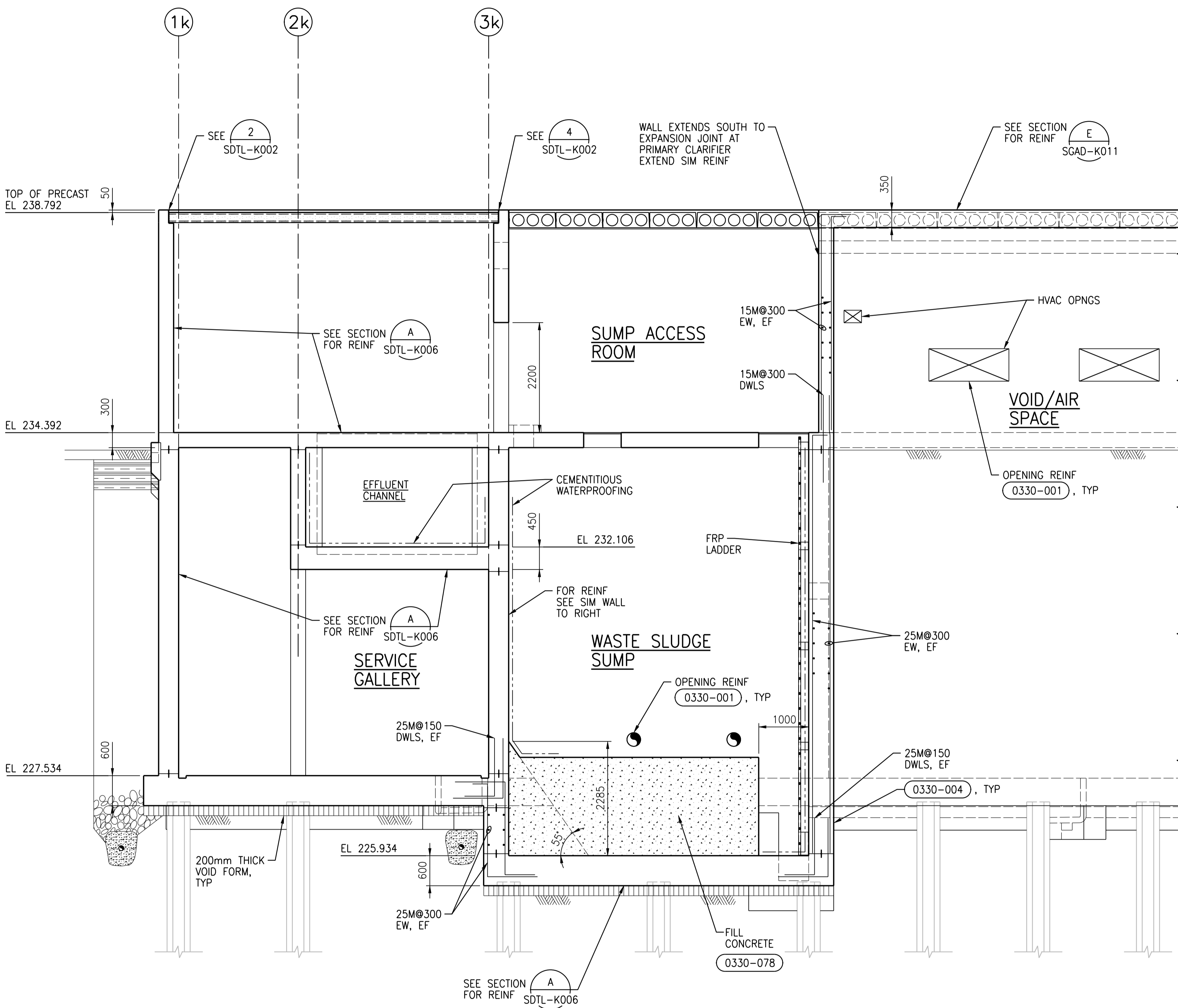
L SECTION 1:50
