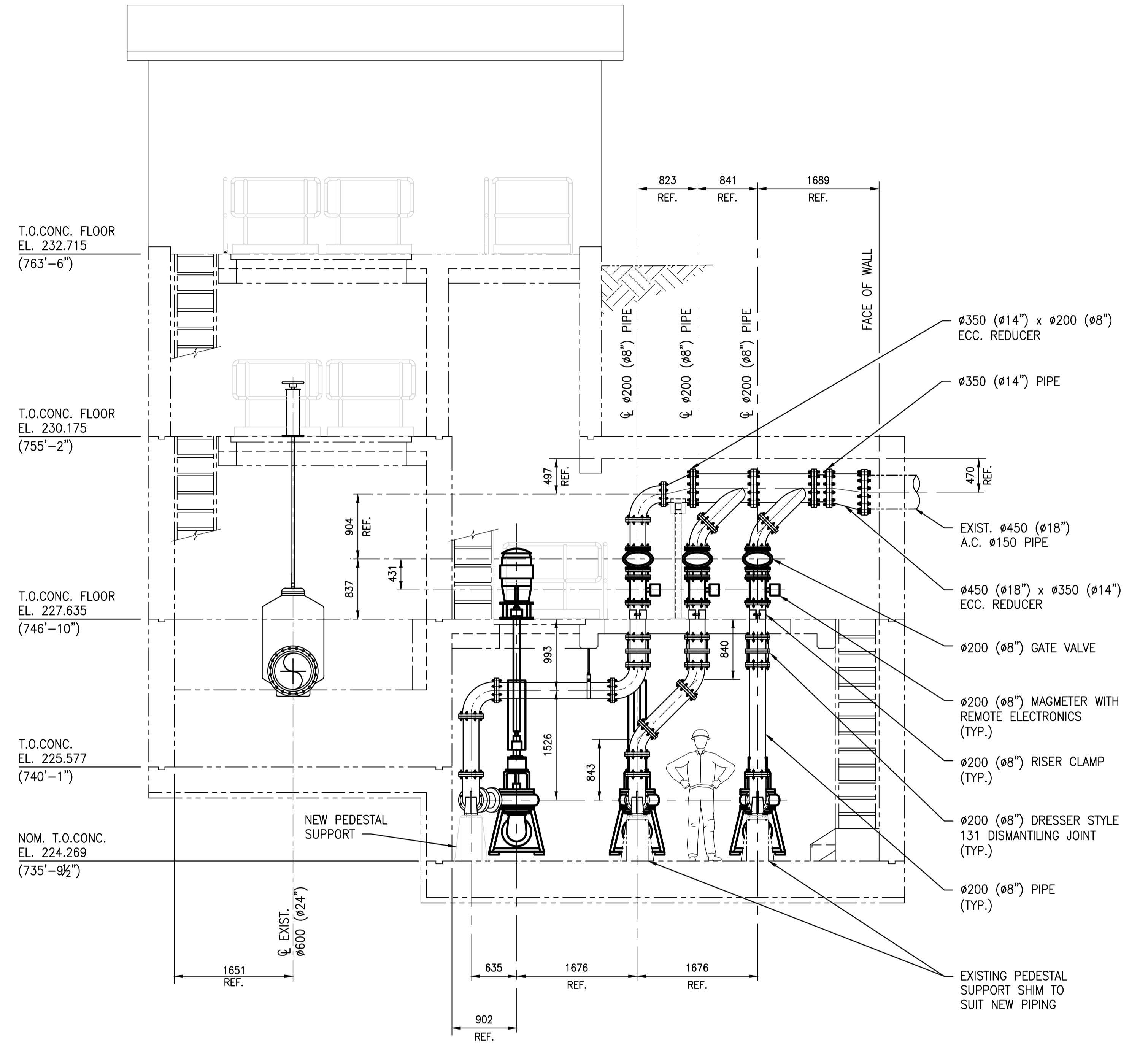
B SECTION M0002 SCALE: 1 : 40
