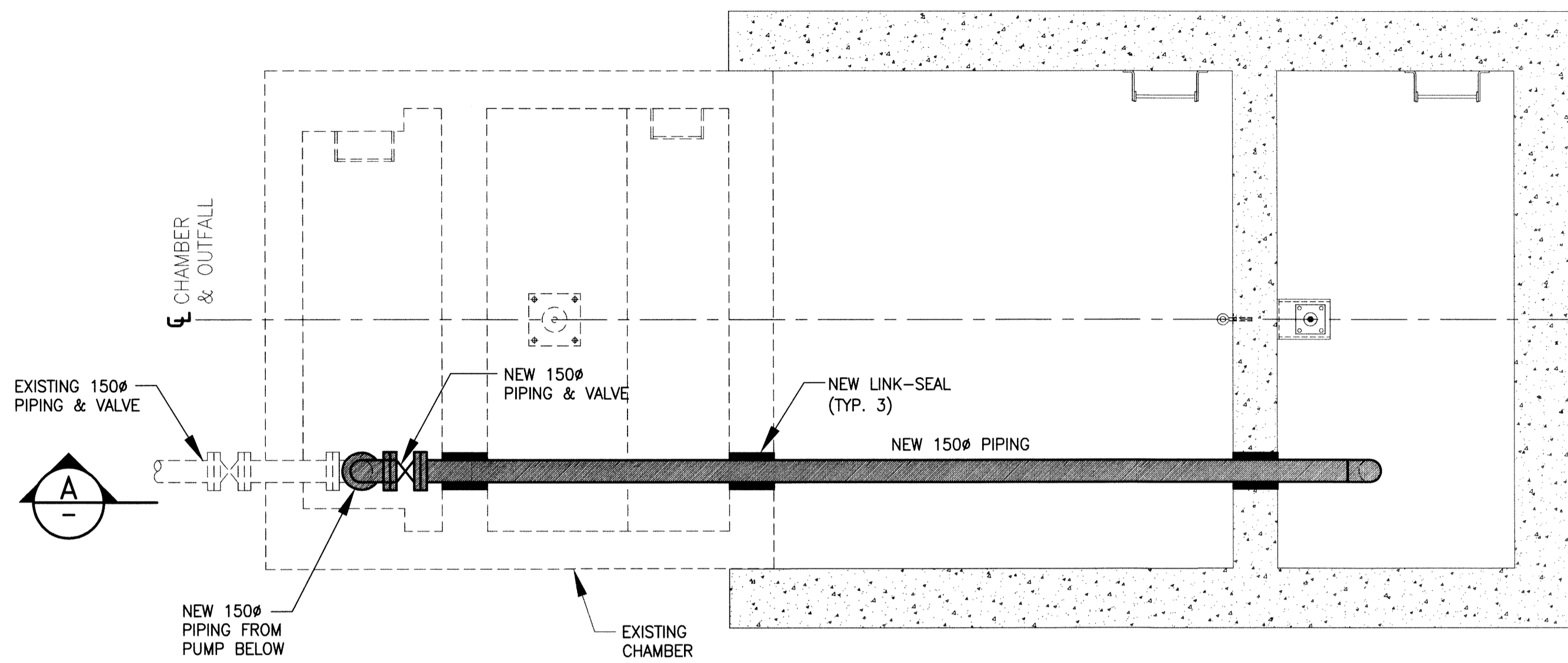
B PLAN - ELEV. - 231.2M SCALE: 1:30
