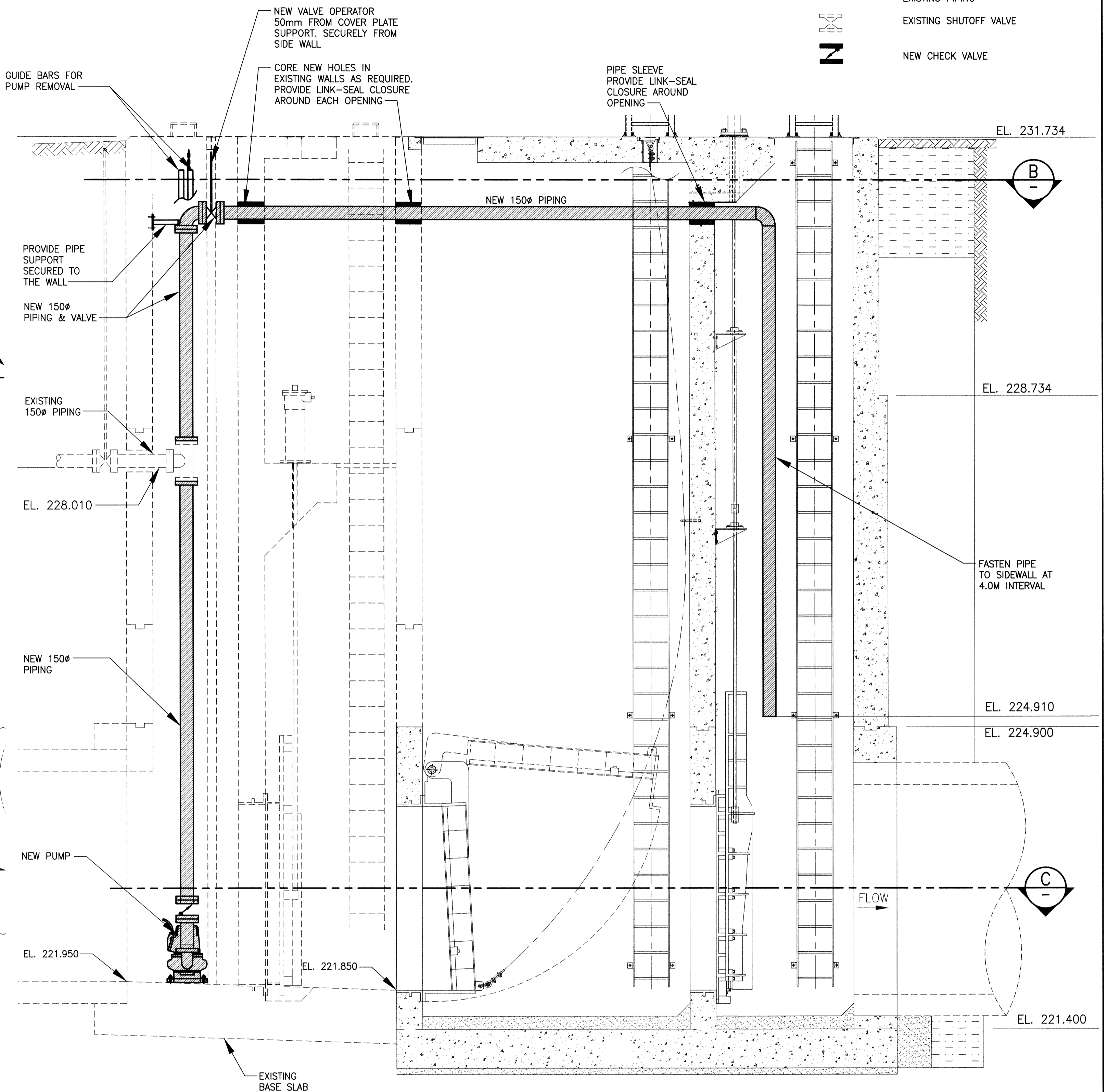
A SECTION SCALE: 1:30
