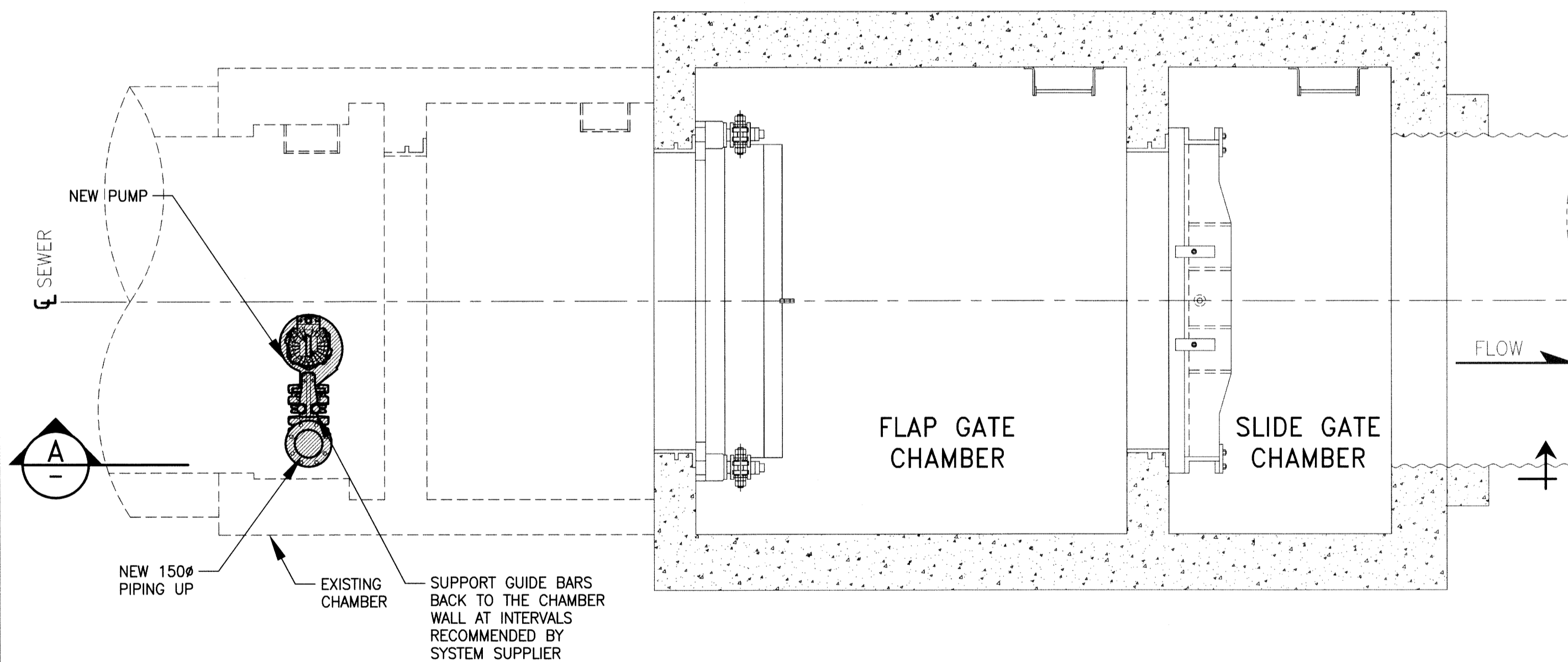
C PLAN - ELEV. - 223M SCALE: 1:30
