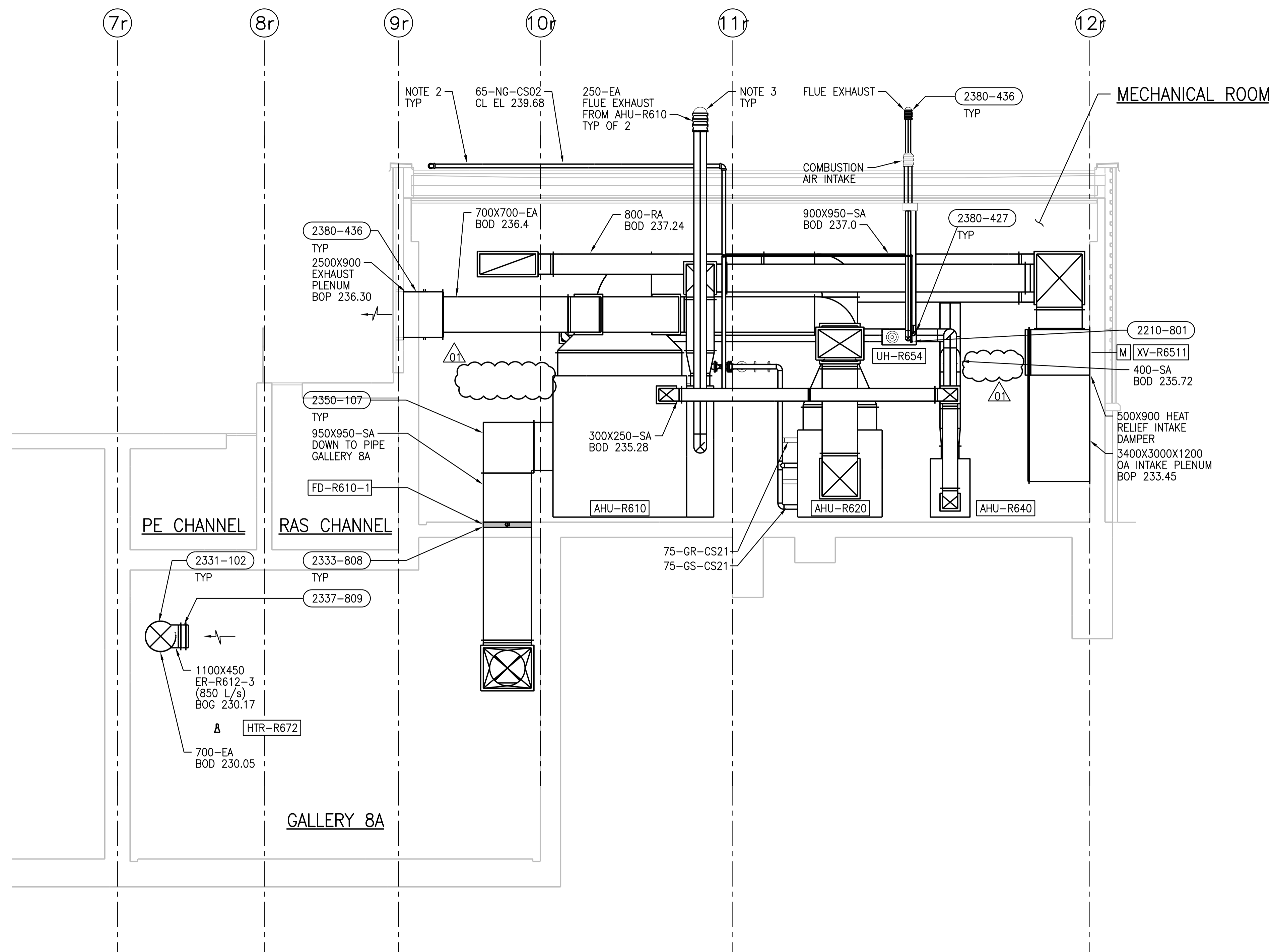
A SECTION 1:50 MGAD-R605 MGAD-R609
