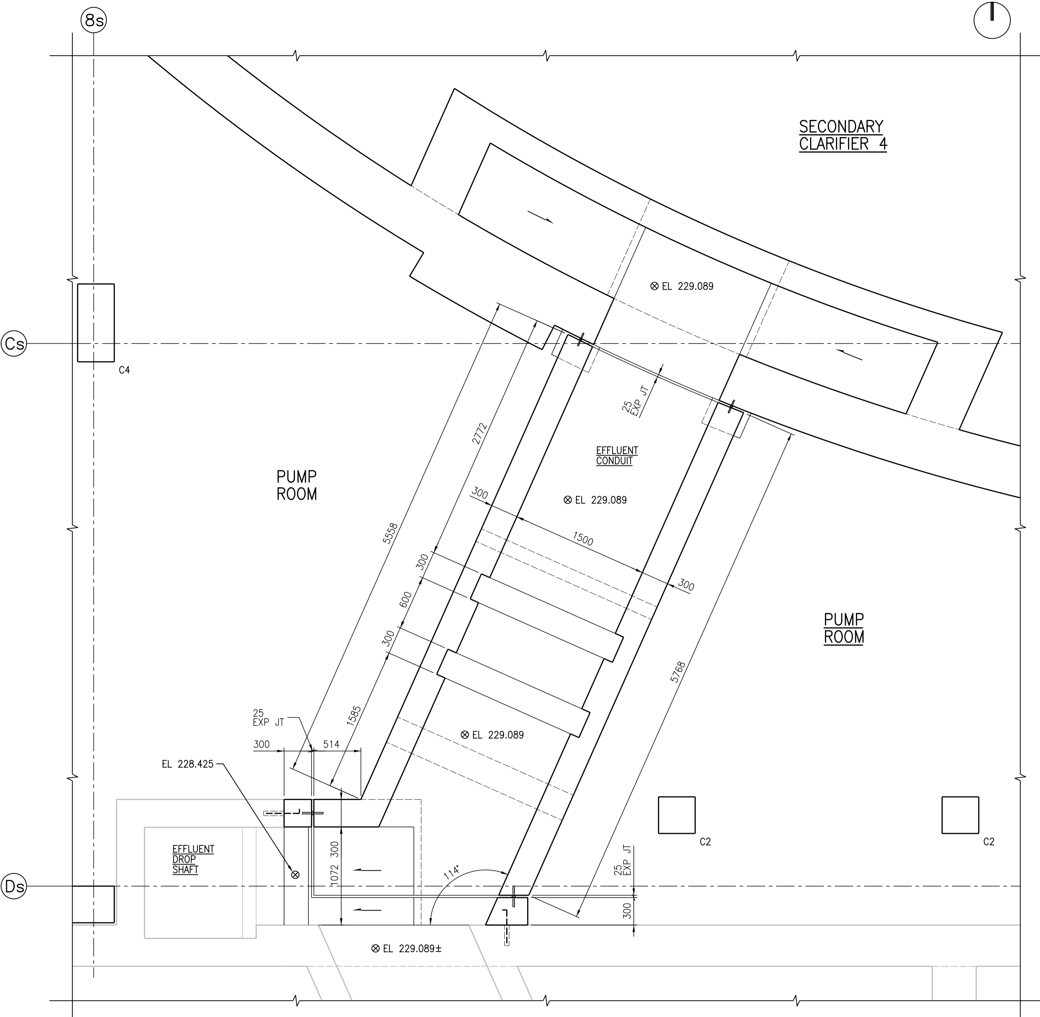
2 DETAIL 1:25 SGAD-S010
