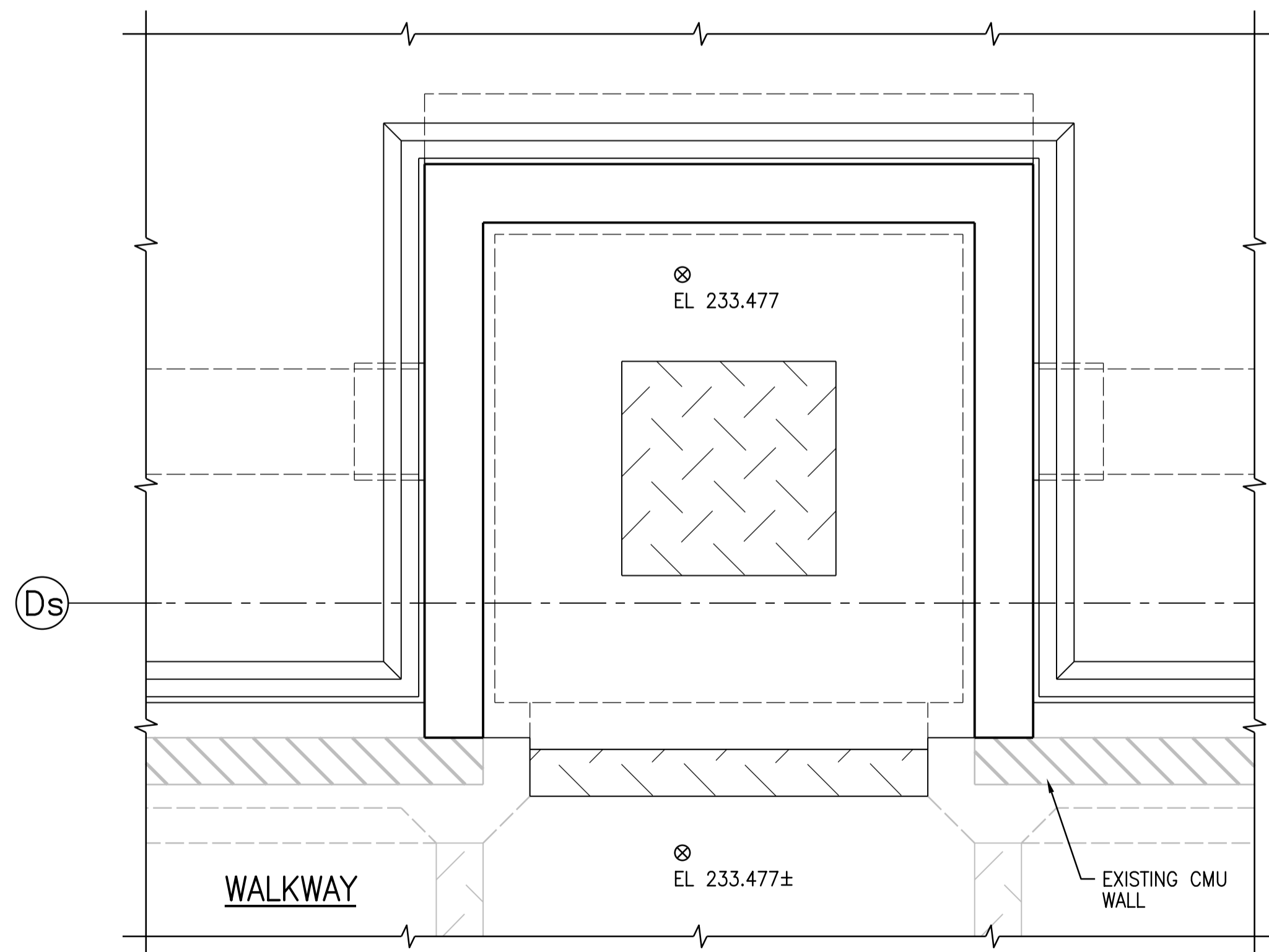
2 DETAIL 1:20 SGAD-S015
