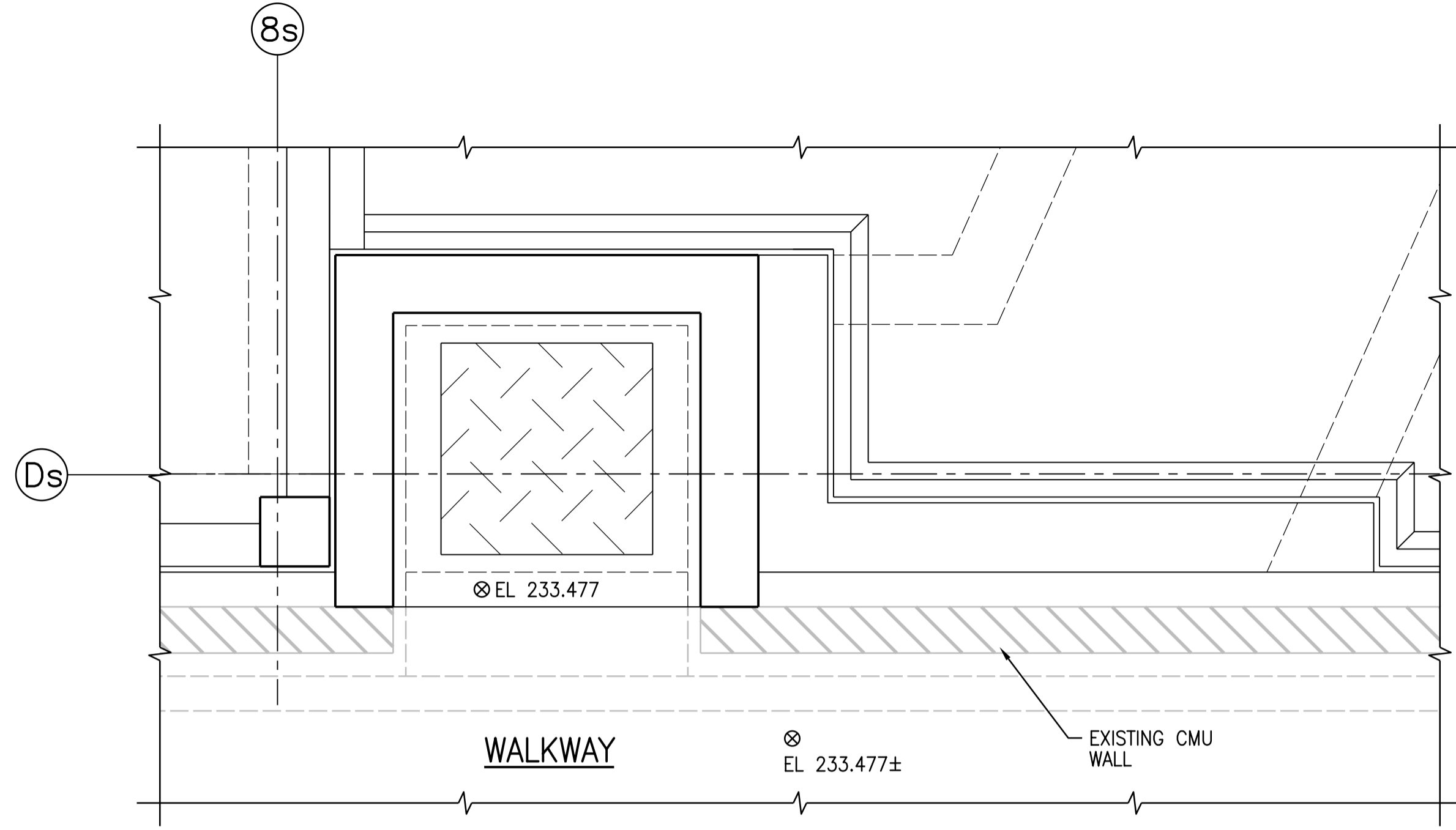
1 DETAIL 1:20 SGAD-S015
