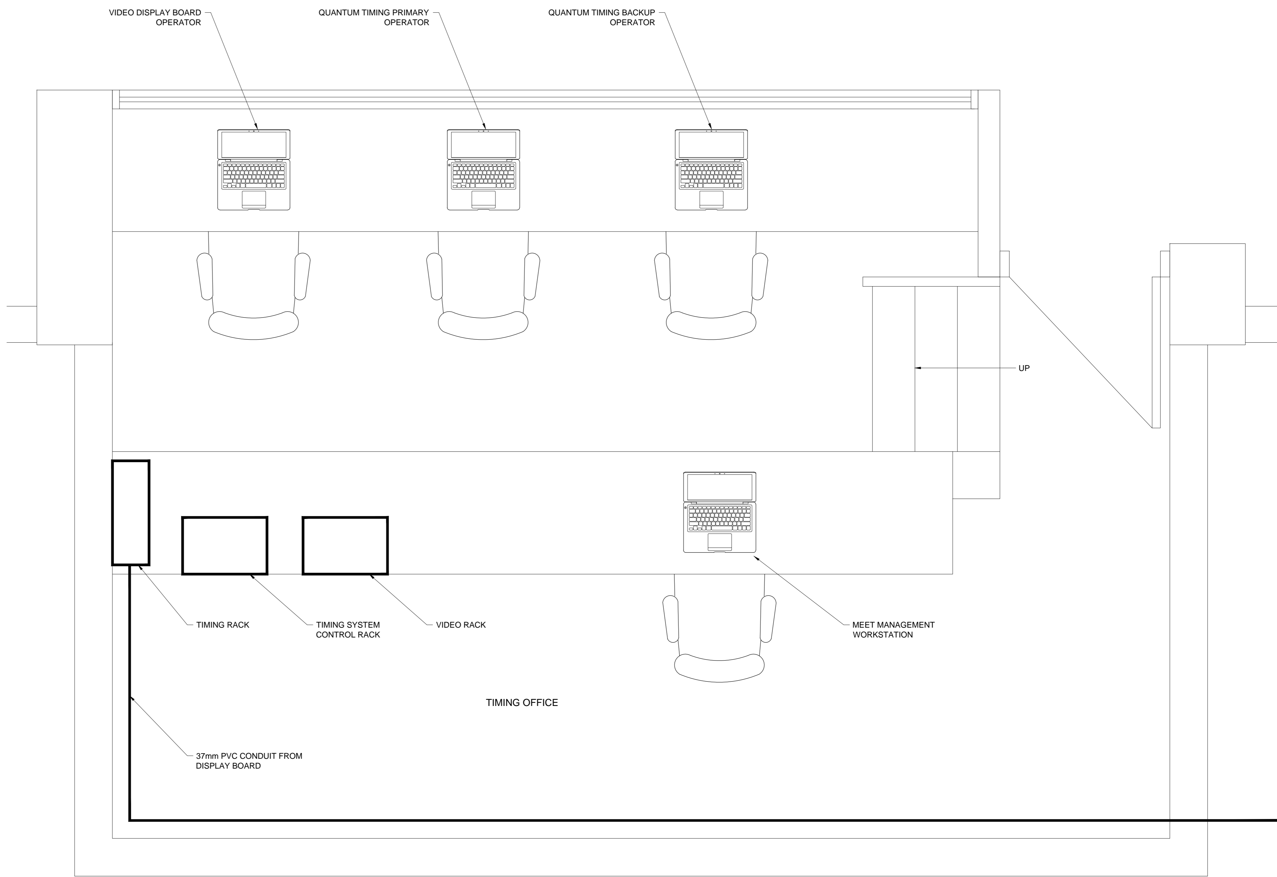
TIMING ROOM LAYOUT 1 1:125 AQ104
