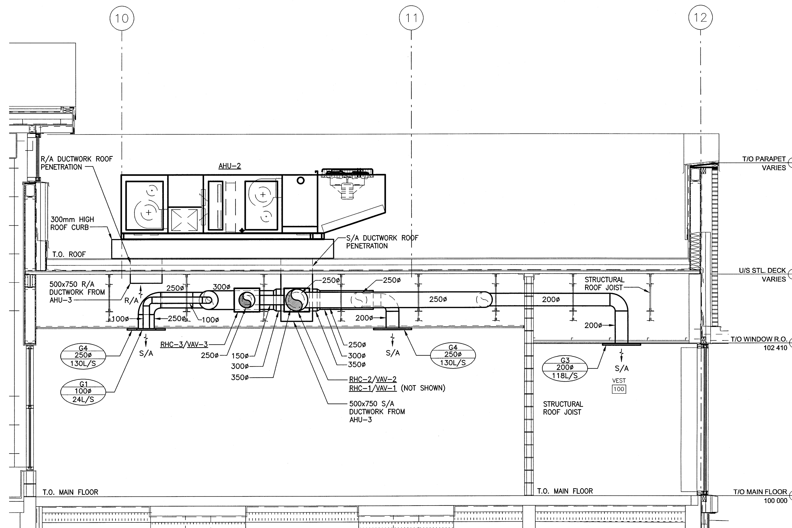
2 AHU-2 AND DUCTWORK DETAILS M3-01 SCALE: N.T.S.
