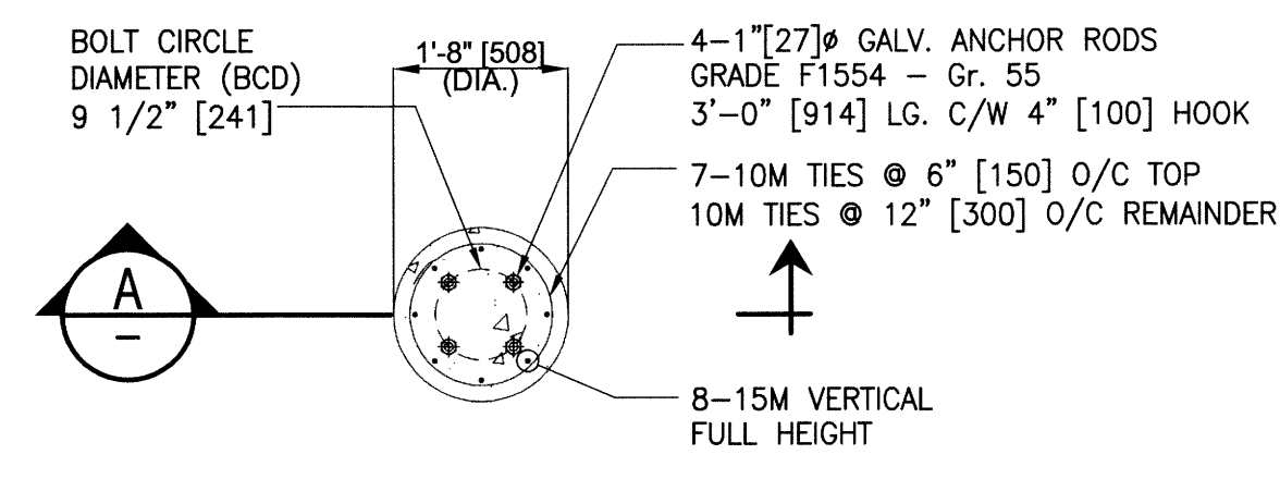
1 DETAIL - PILE 'P1' SCALE: N.T.S.
