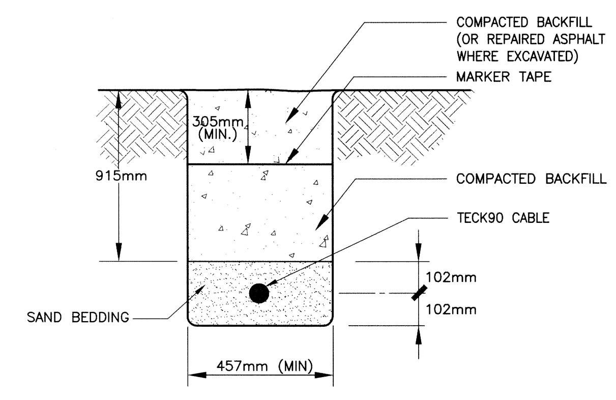
3 TRENCH DETAIL SCALE: N.T.S.
