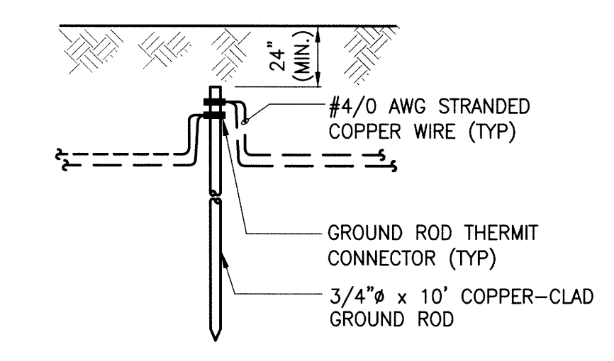
4 GROUND ROD DETAIL SCALE: N.T.S.
