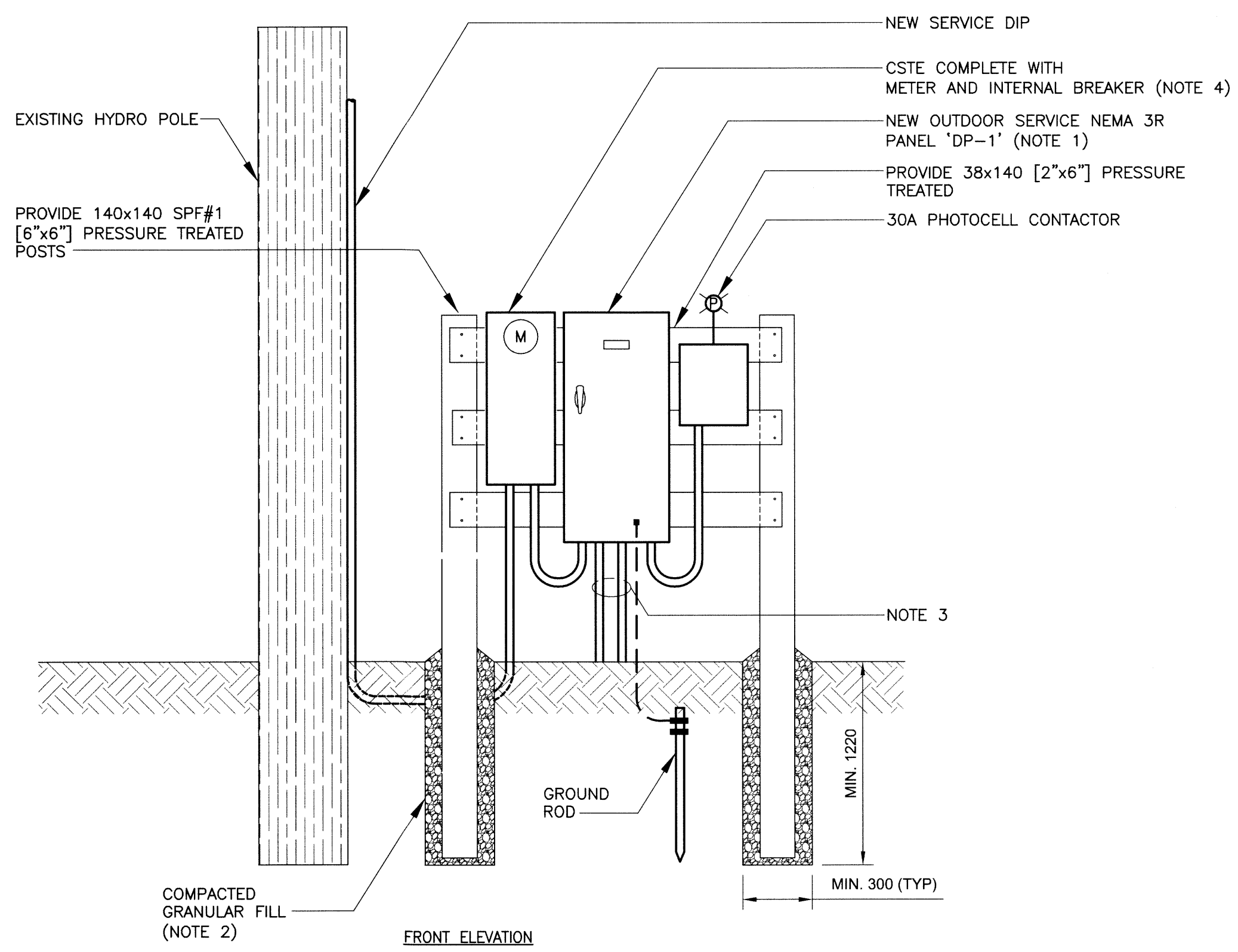
2 PANEL DP-1 MOUNTING DETAIL SCALE: N.T.S. (NOTE 4)
