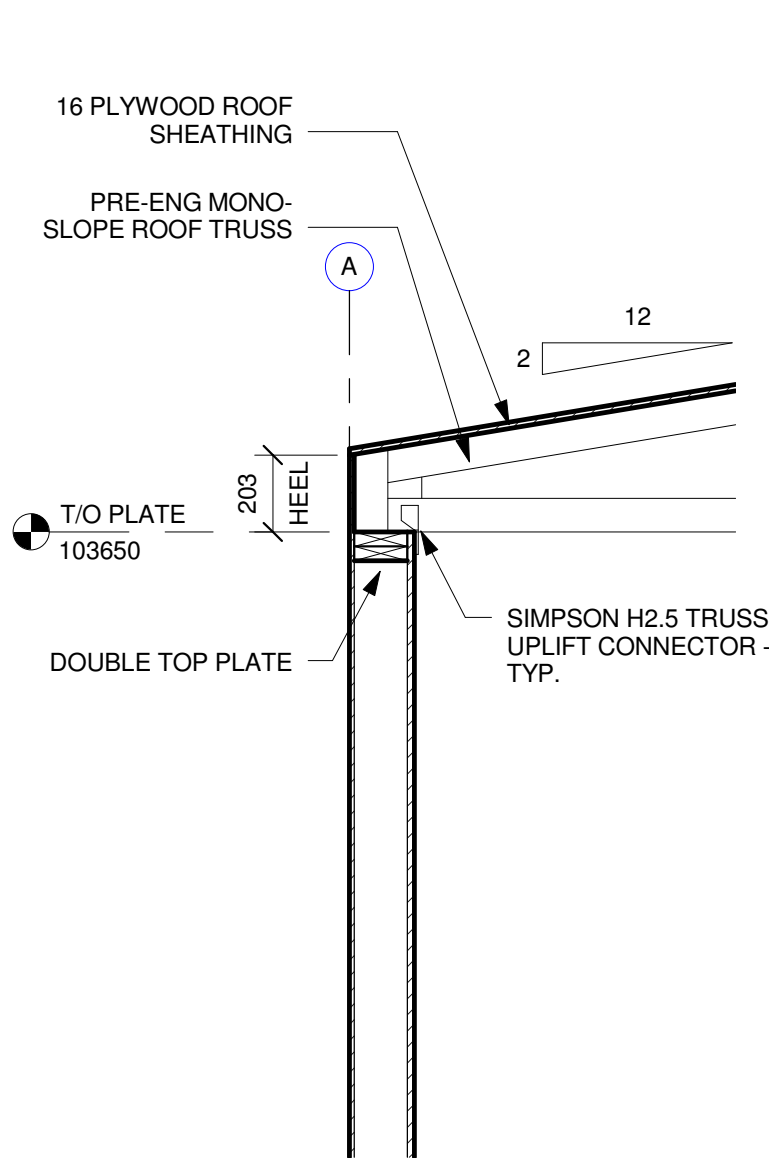
1 SECTION S501 1 : 20
