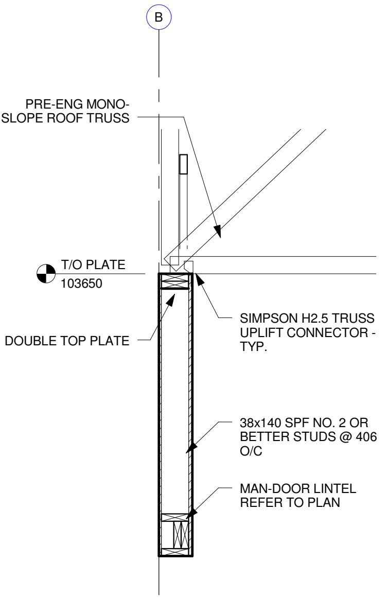
2 SECTION S501 1 : 20
