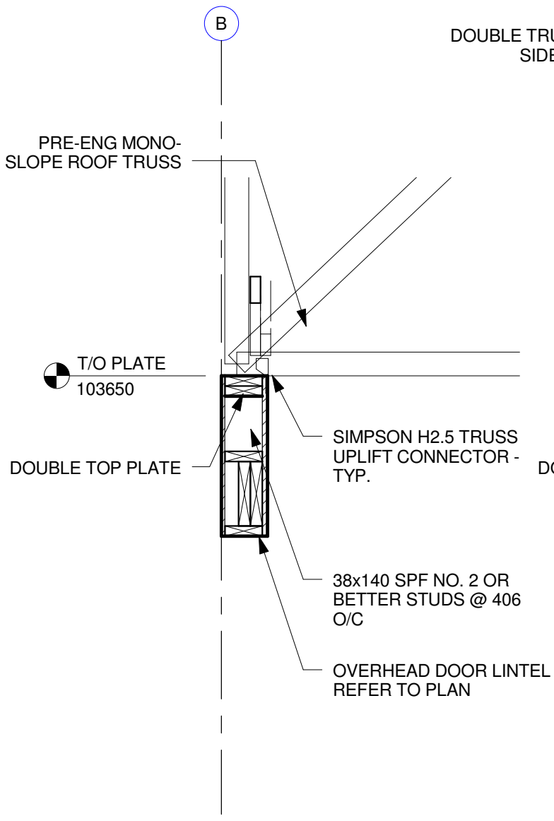
3 SECTION S501 1 : 20
