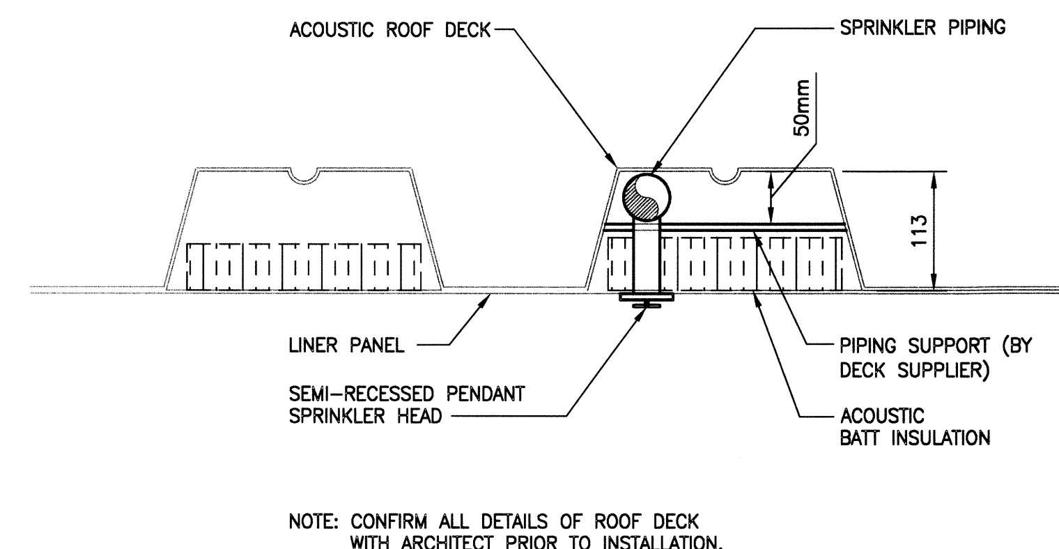
4 SPRINKLER PIPING INSTALLATION DETAIL IN SPLASH PAD SCALE: N.T.S.
