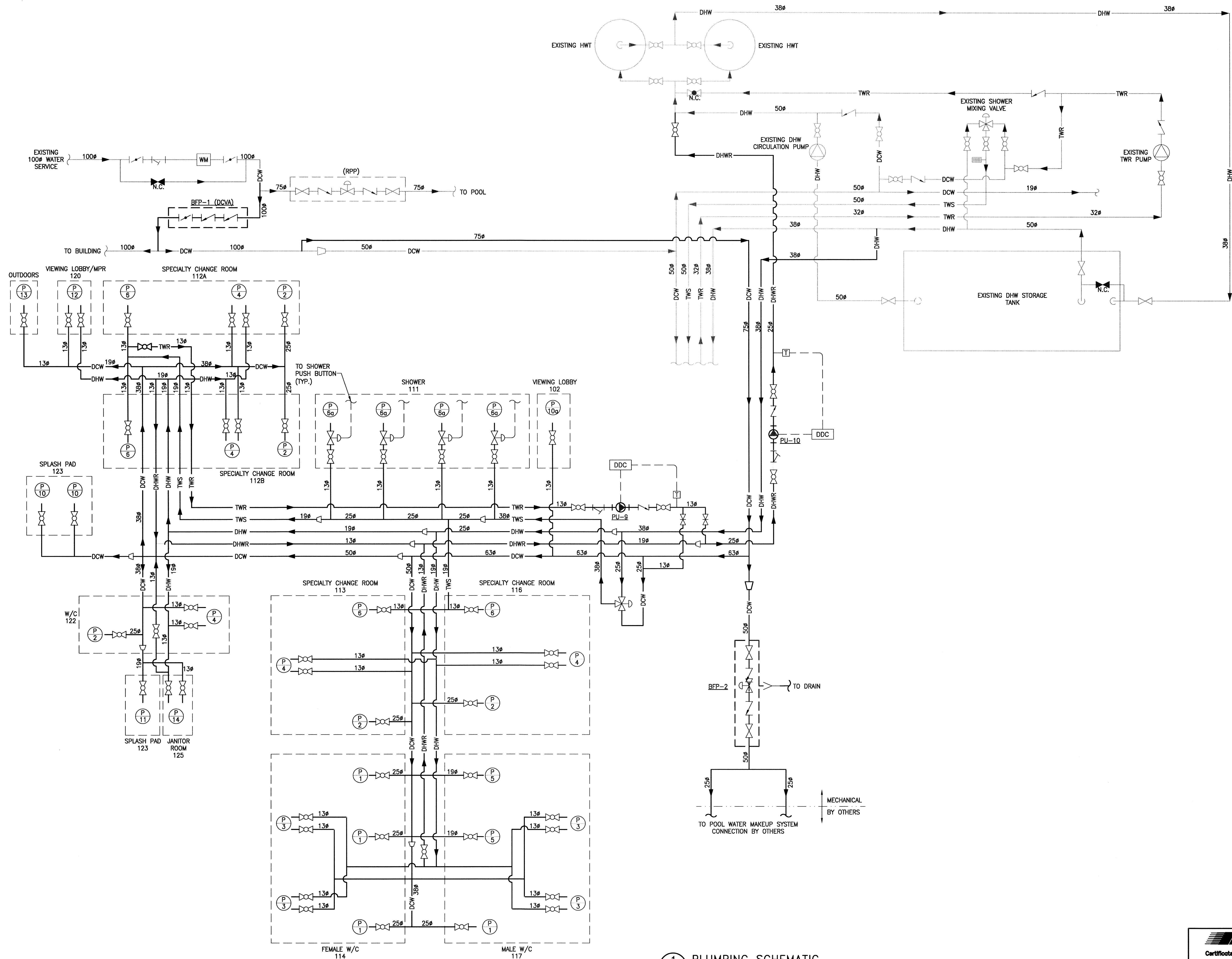
1 PLUMBING SCHEMATIC SCALE: N.T.S.
