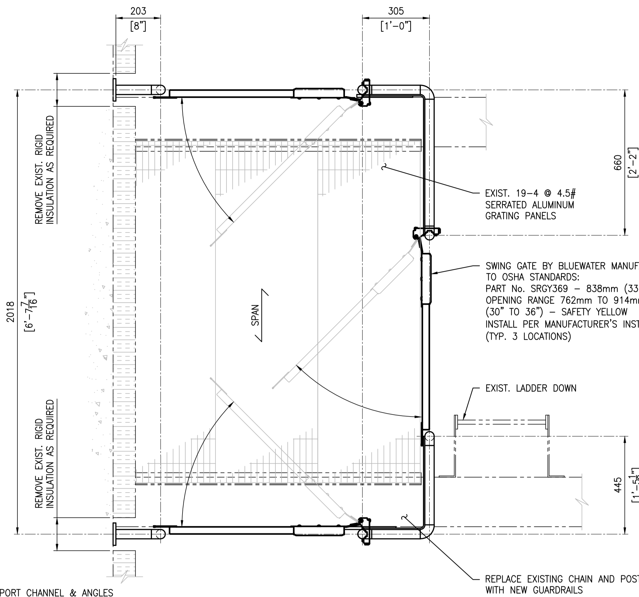
PLAN - GUARDRAIL SCALE: 1 : 10
