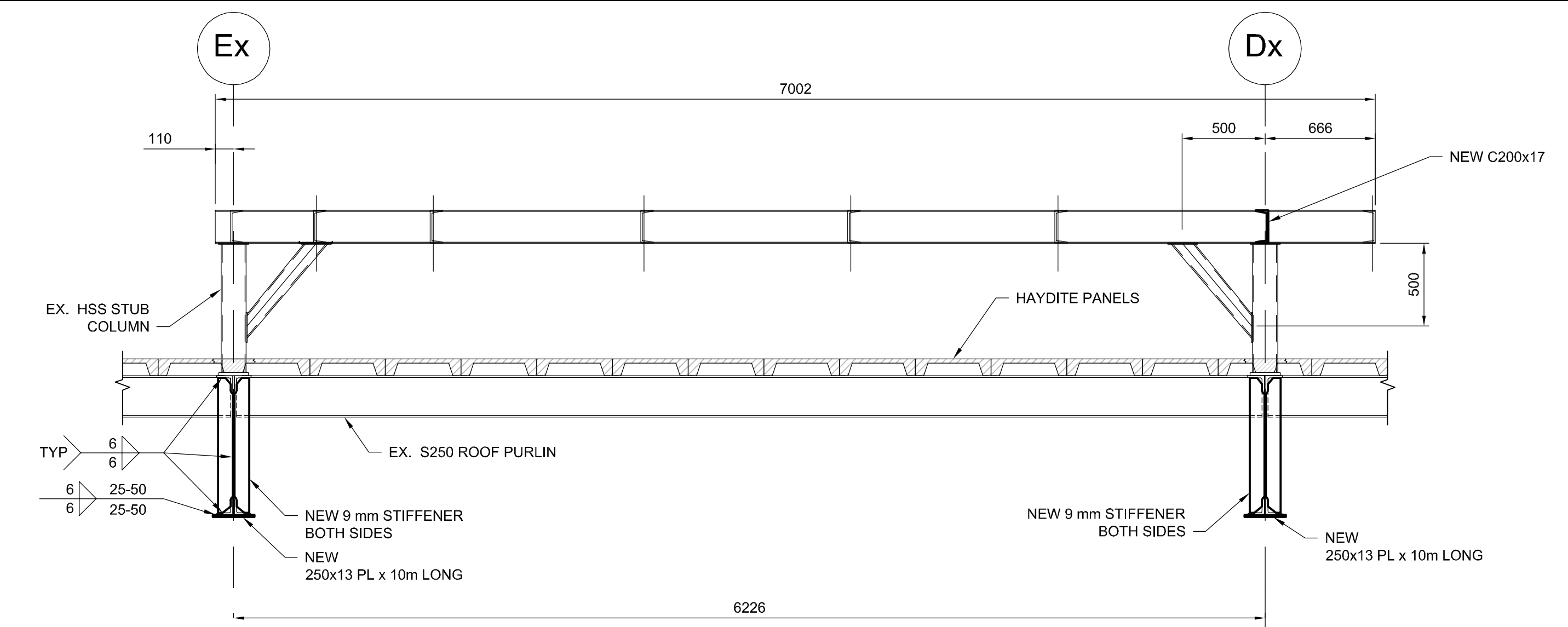
F SECTION 1:25
