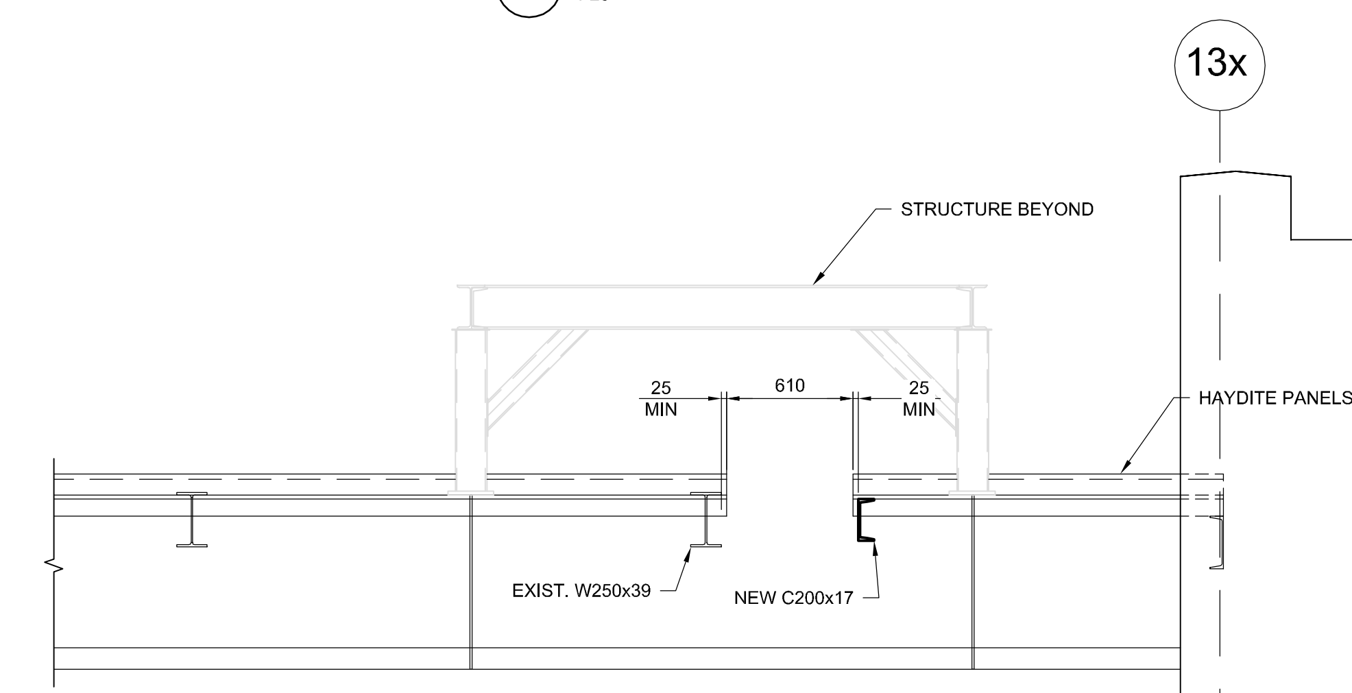
H SECTION 1:25
