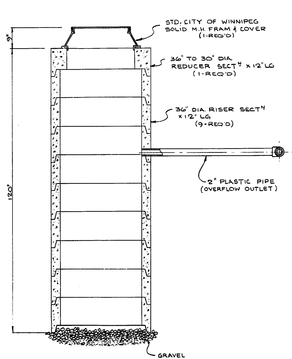
SECTION A-A
