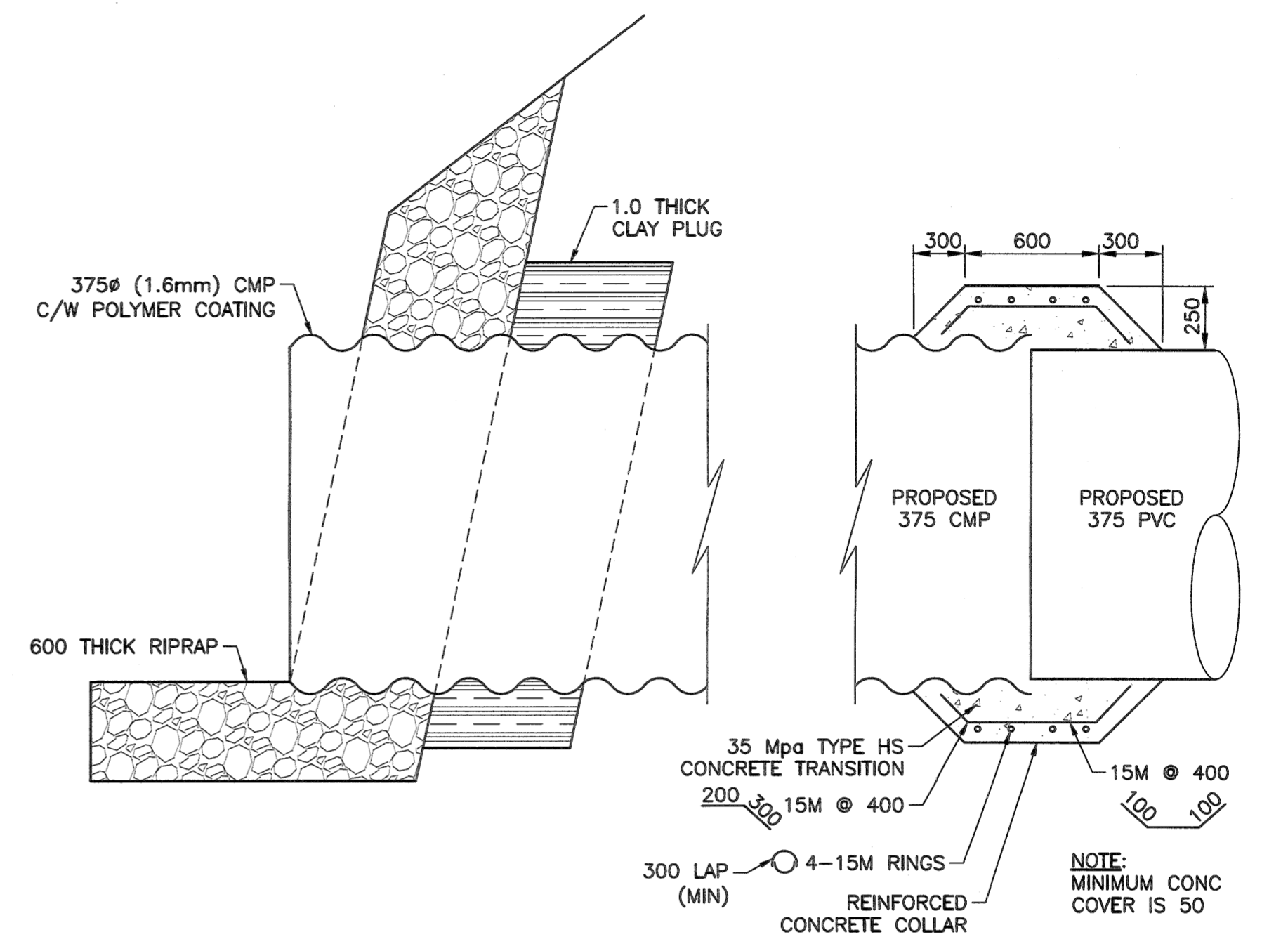
CONCRETE COLLAR AND END SECTION DETAIL SCALE: N.T.S.
