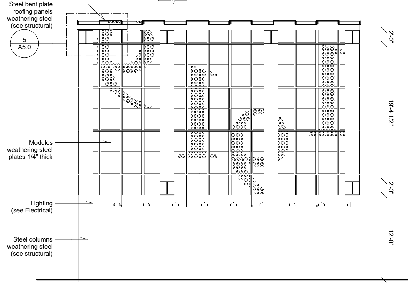
1 Section Scale: 1/8" = 1'-0"
