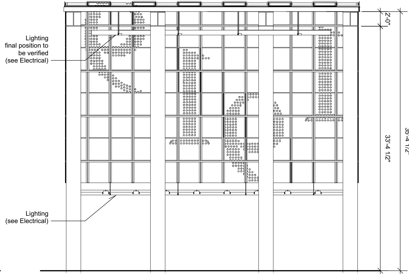
2 Section Scale: 1/8" = 1'-0"
