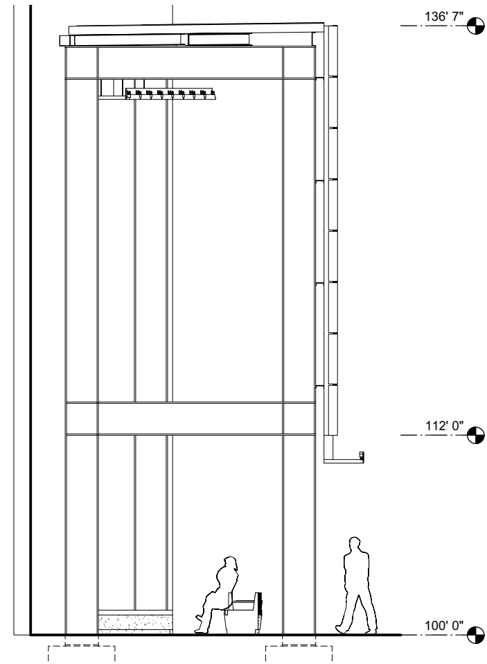
4 North elevation Scale: 1/8" = 1'-0"
