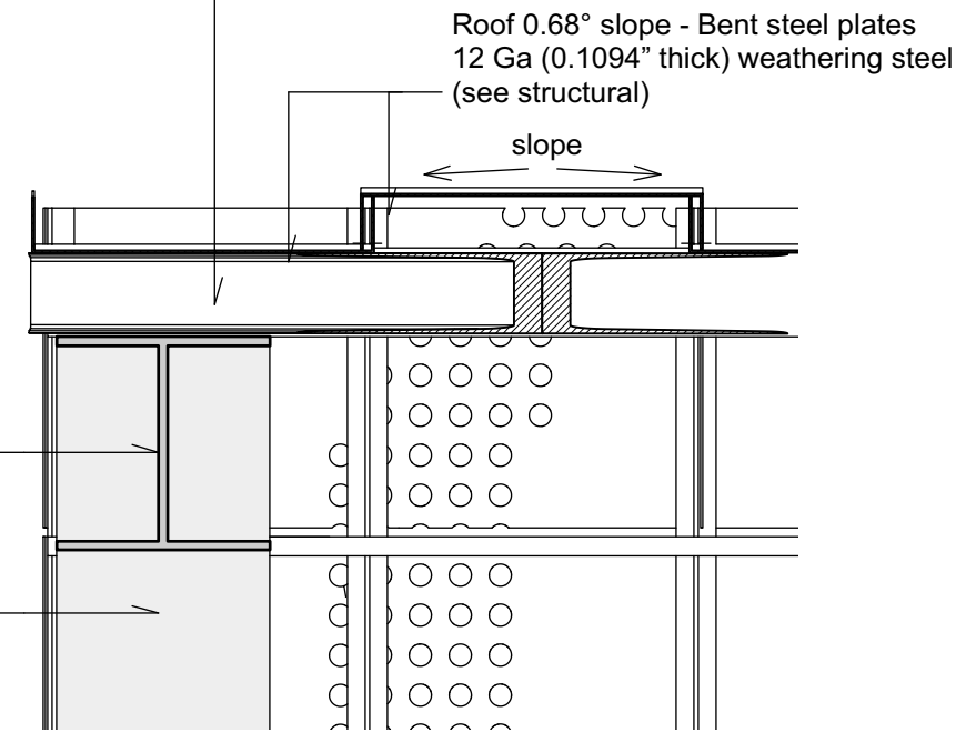
5 Detail 5 Scale: 1/2" = 1'-0"
