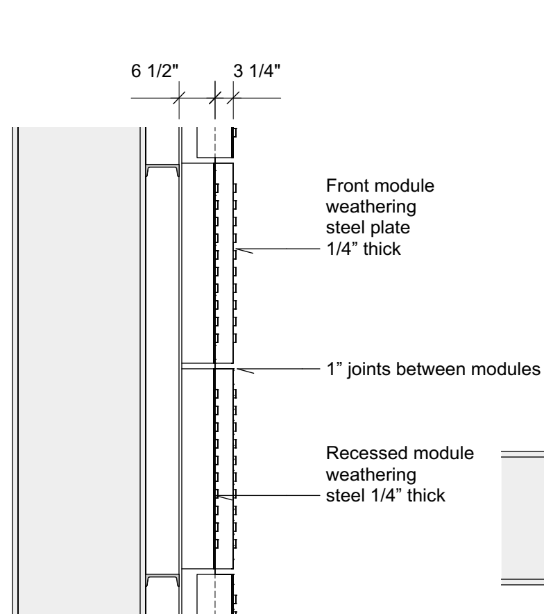
4 Detail 4 Scale: 1/2" = 1'-0"
