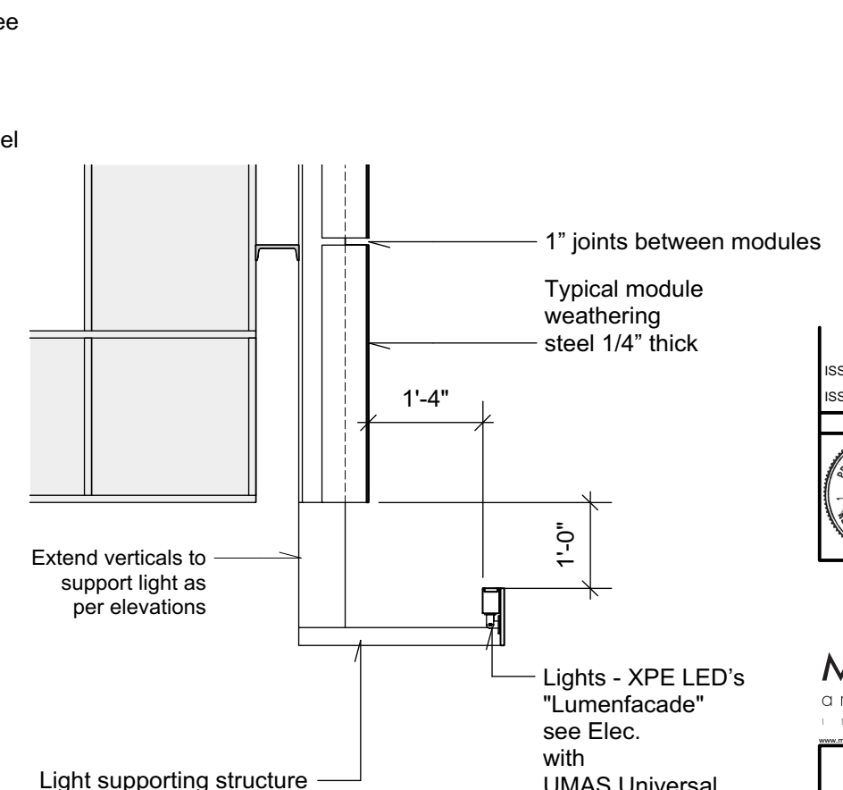
6 Detail 6 Scale: 1/2" = 1'-0"
