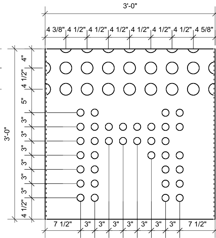
2 Module G08 Scale: 1" = 1'-0"
