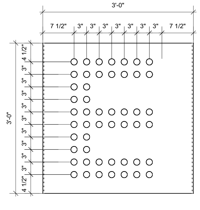
4 Module G10 Scale: 1" = 1'-0"
