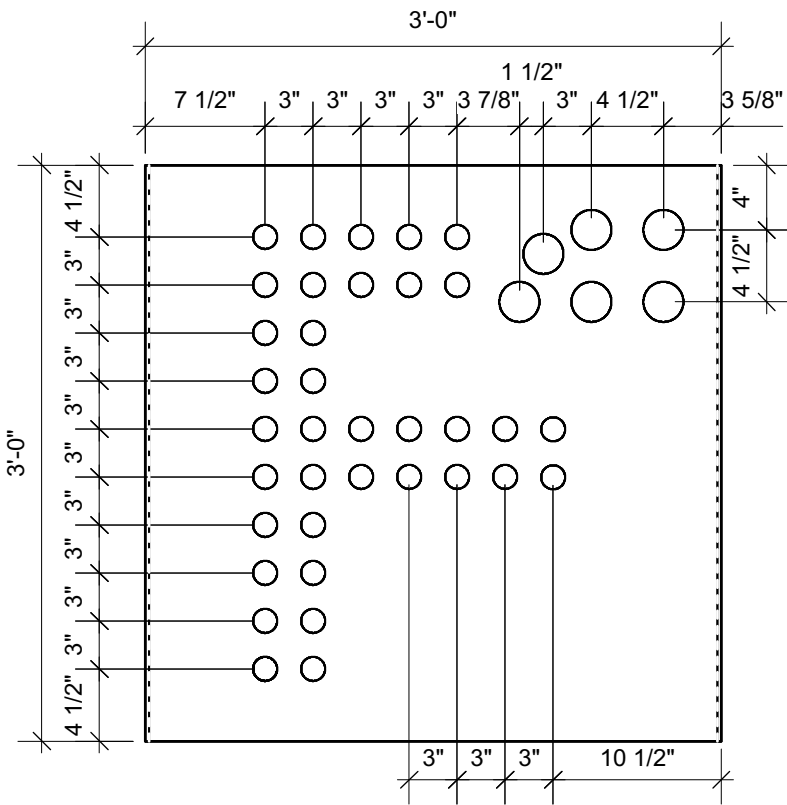
1 Module G07 Scale: 1" = 1'-0"
