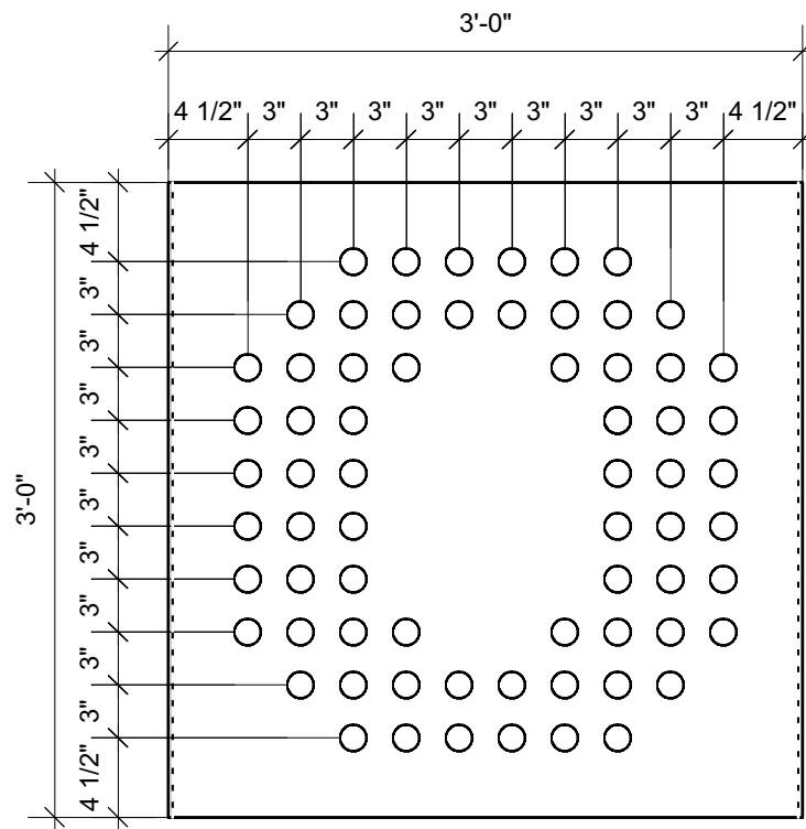
6 Module G12 Scale: 1" = 1'-0"
