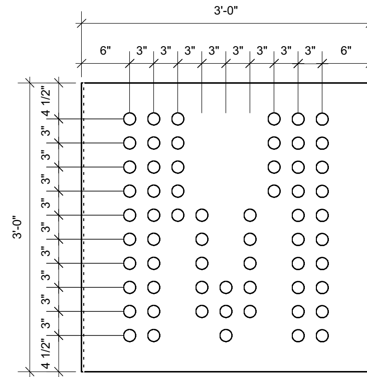
7 Module G13 Scale: 1" = 1'-0"
