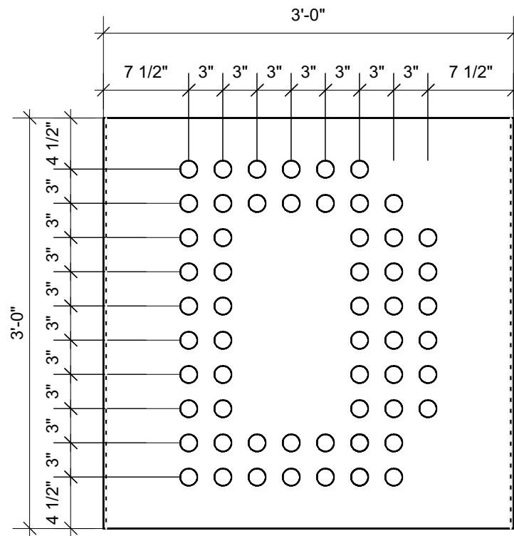
5 Module G11 Scale: 1" = 1'-0"
