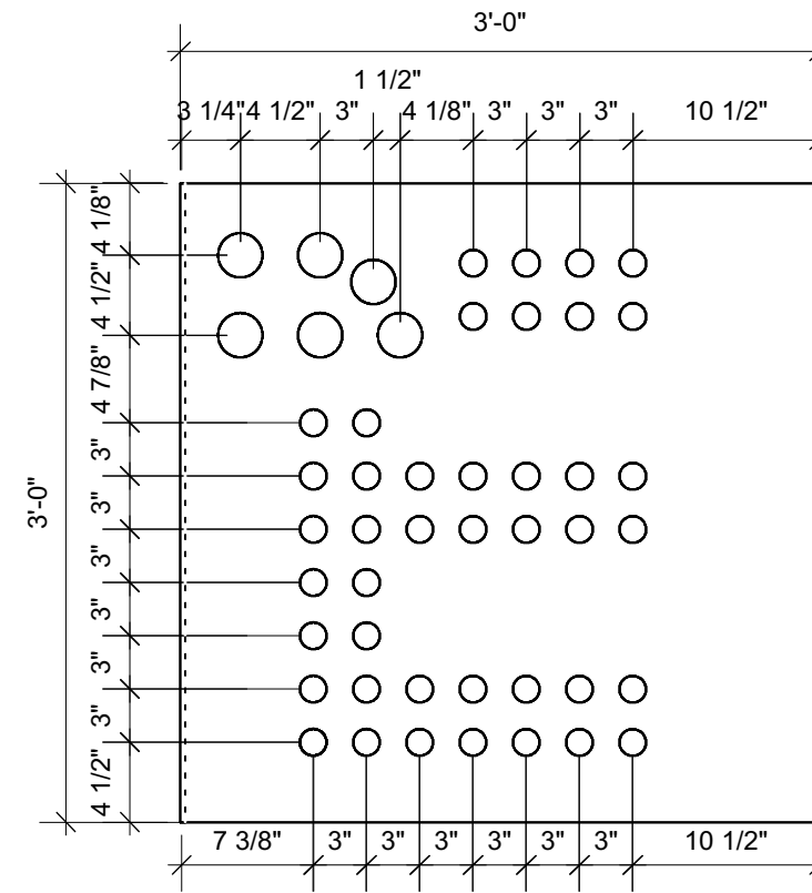
3 Module G09 Scale: 1" = 1'-0"
