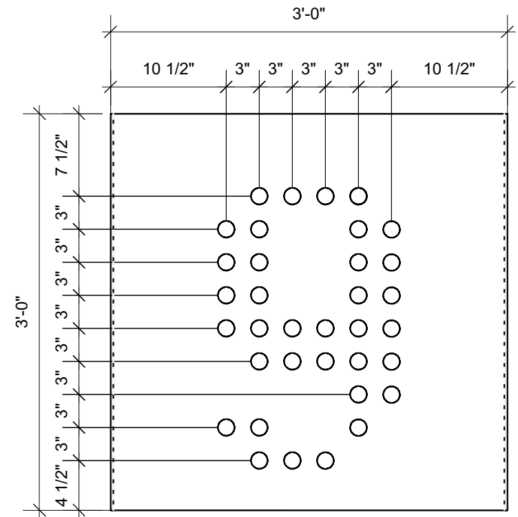
4 Module H04 Scale: 1" = 1'-0"
