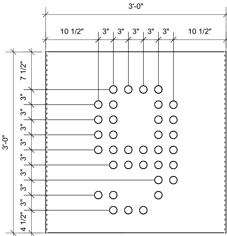
2 Module H02 Scale: 1" = 1'-0"
