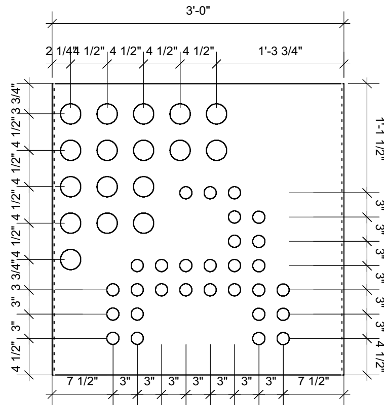
6 Module H06 Scale: 1" = 1'-0"
