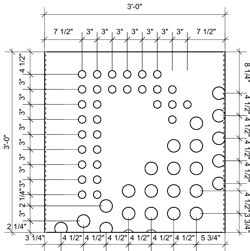
5 Module H05 Scale: 1" = 1'-0"
