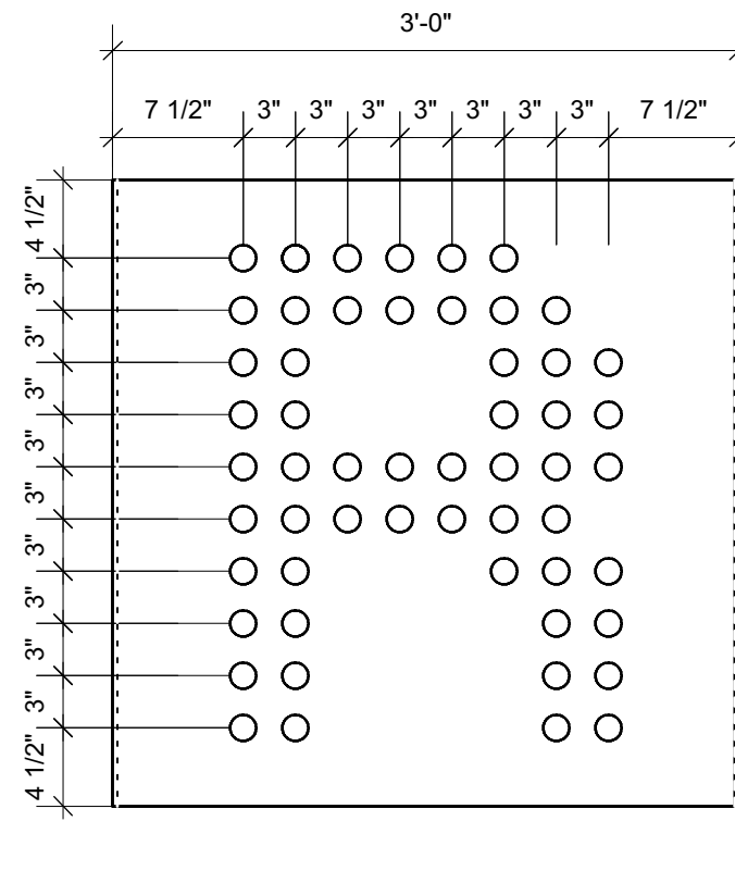
7 Module H07 Scale: 1" = 1'-0"
