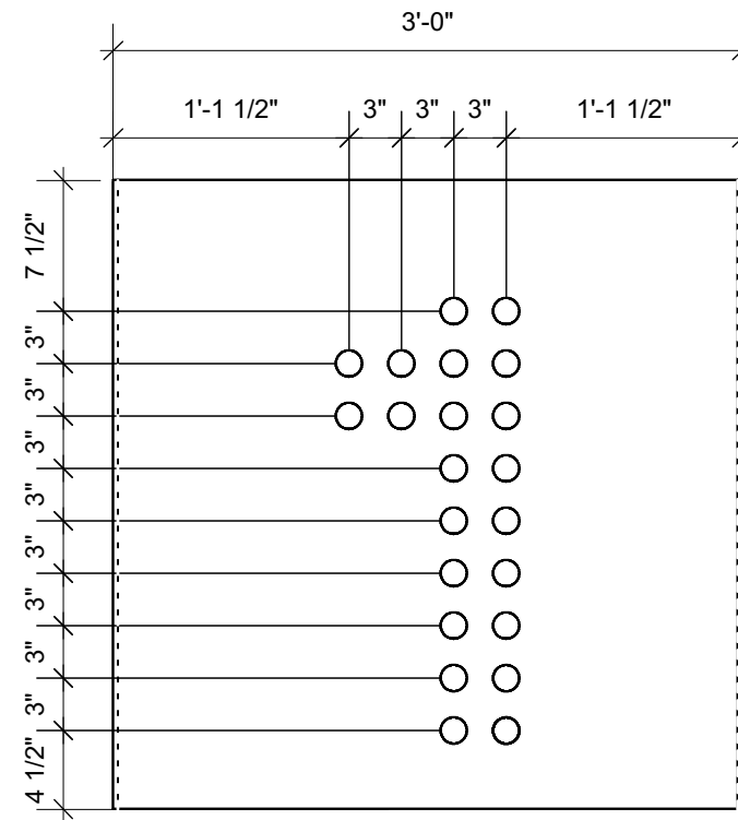
3 Module H03 Scale: 1" = 1'-0"
