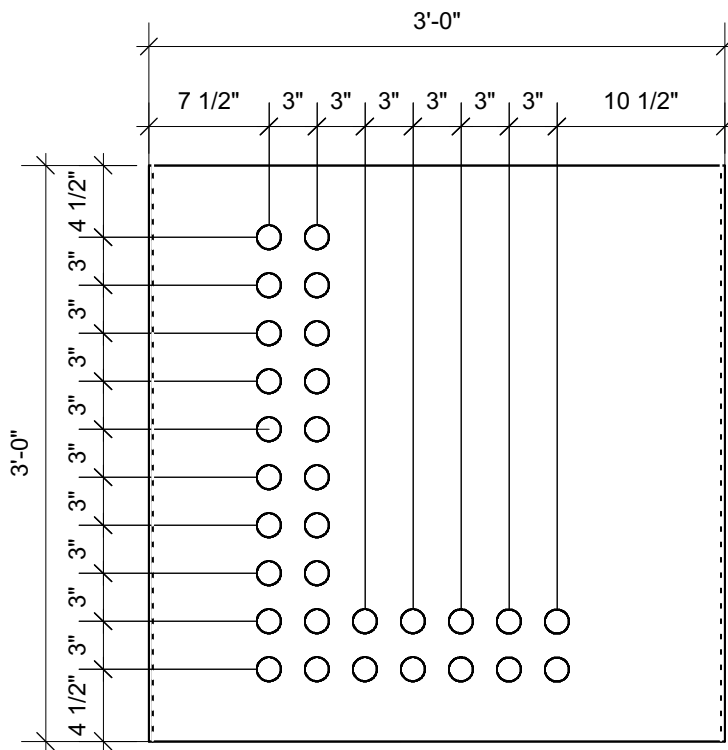
6 Module H13 Scale: 1" = 1'-0"
