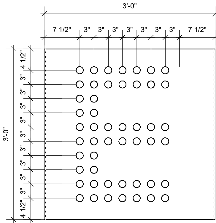
2 Module H09 Scale: 1" = 1'-0"
