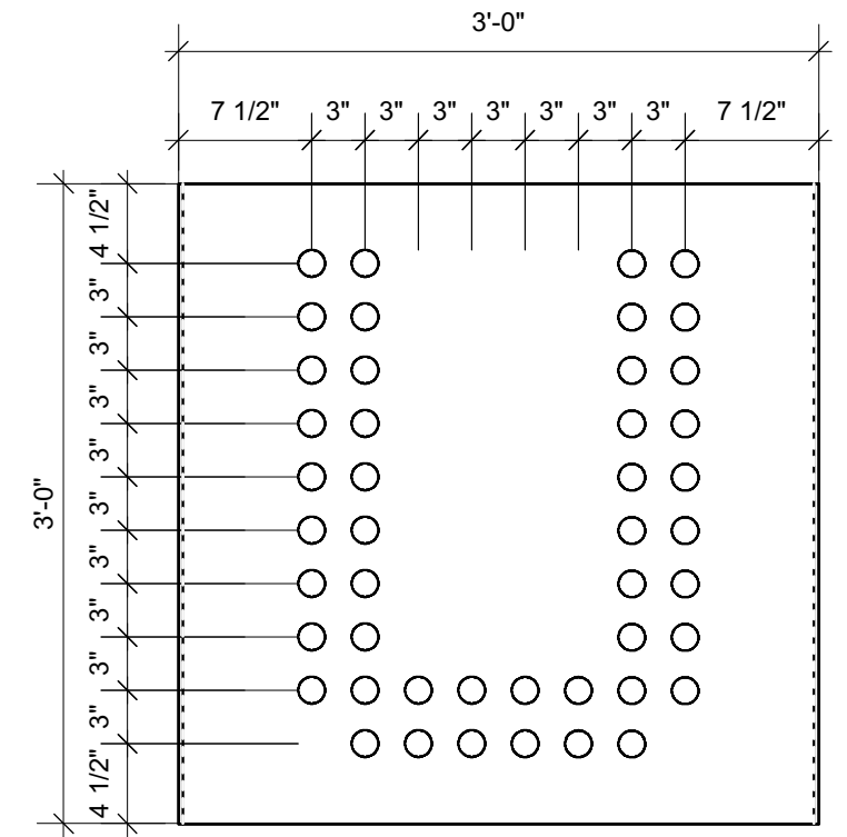
4 Module H11 Scale: 1" = 1'-0"
