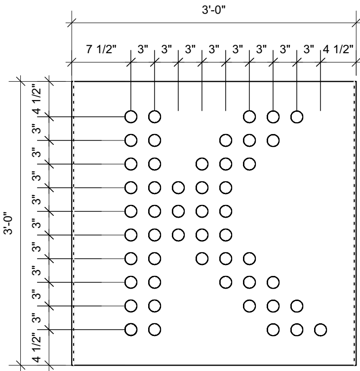
1 Module H08 Scale: 1" = 1'-0"
