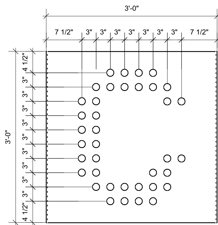
6 Module A06 Scale: 1" = 1'-0"
