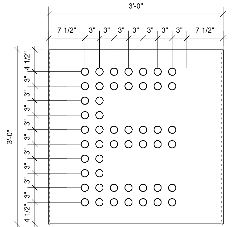
4 Module A04 Scale: 1" = 1'-0"
