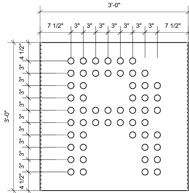
2 Module A02 Scale: 1" = 1'-0"
