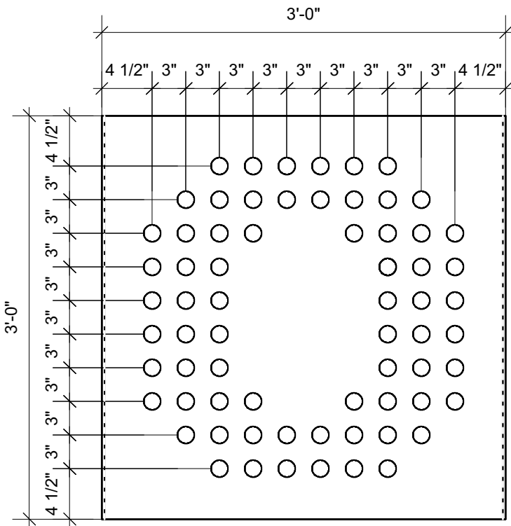
1 Module A01 Scale: 1" = 1'-0"
