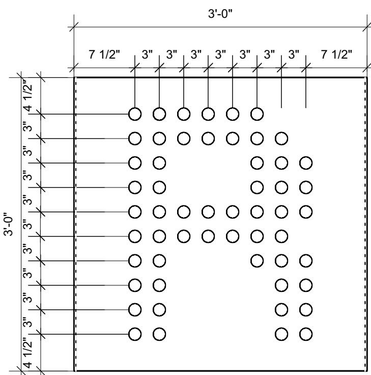
5 Module A05 Scale: 1" = 1'-0"
