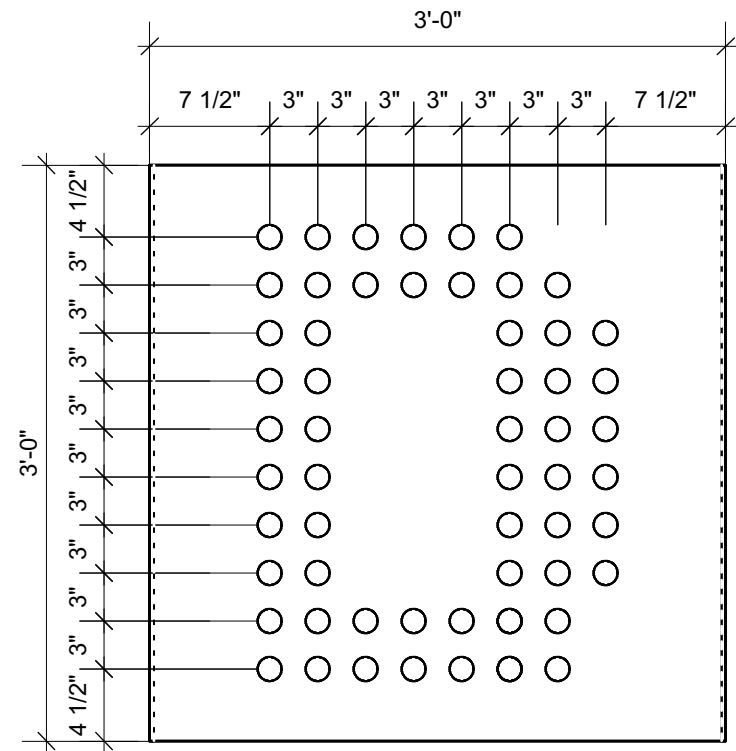
3 Module A03 Scale: 1" = 1'-0"
