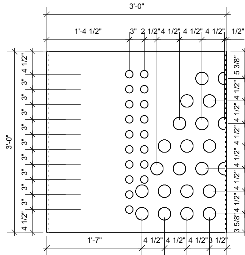
3 Module A10 Scale: 1" = 1'-0"
