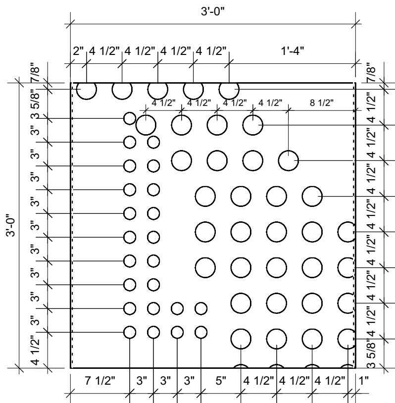
5 Module A12 Scale: 1" = 1'-0"
