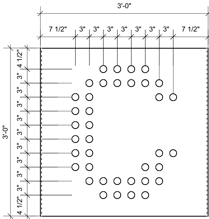
2 Module A09 Scale: 1" = 1'-0"
