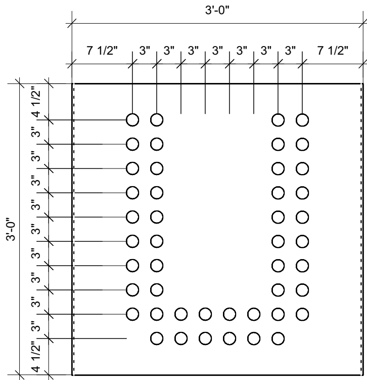
1 Module A08 Scale: 1" = 1'-0"
