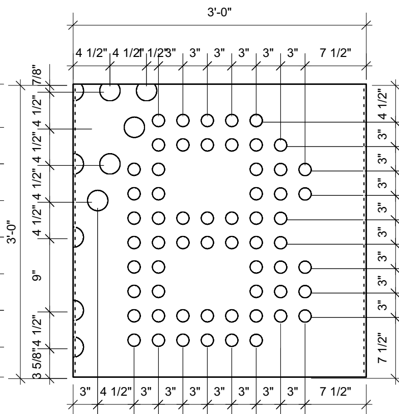
4 Module A11 Scale: 1" = 1'-0"
