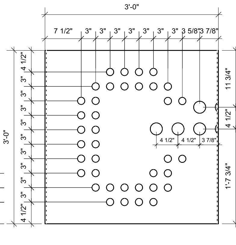
7 Module B01 Scale: 1" = 1'-0"
