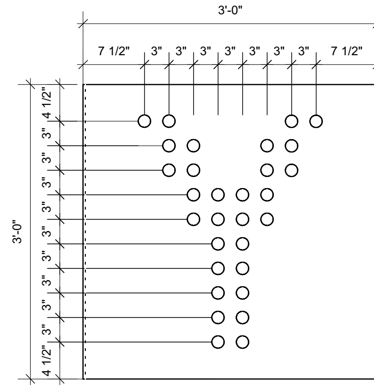
3 Module B04 Scale: 1" = 1'-0"
