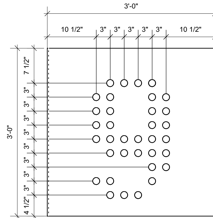
7 Module B08 Scale: 1" = 1'-0"
