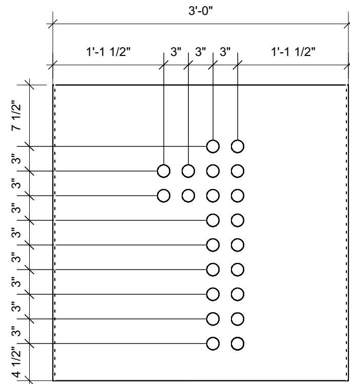
6 Module B07 Scale: 1" = 1'-0"
