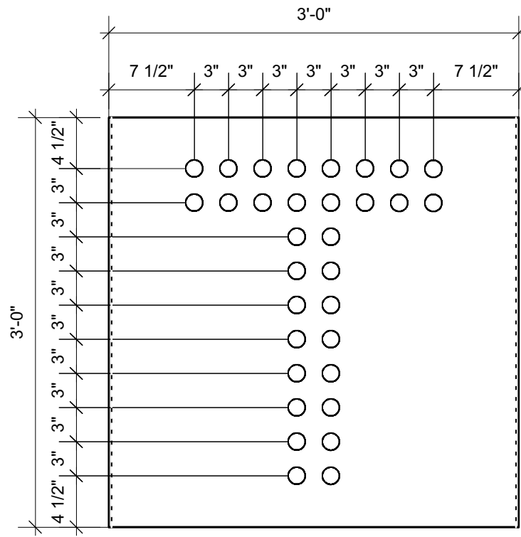
2 Module B03 Scale: 1" = 1'-0"
