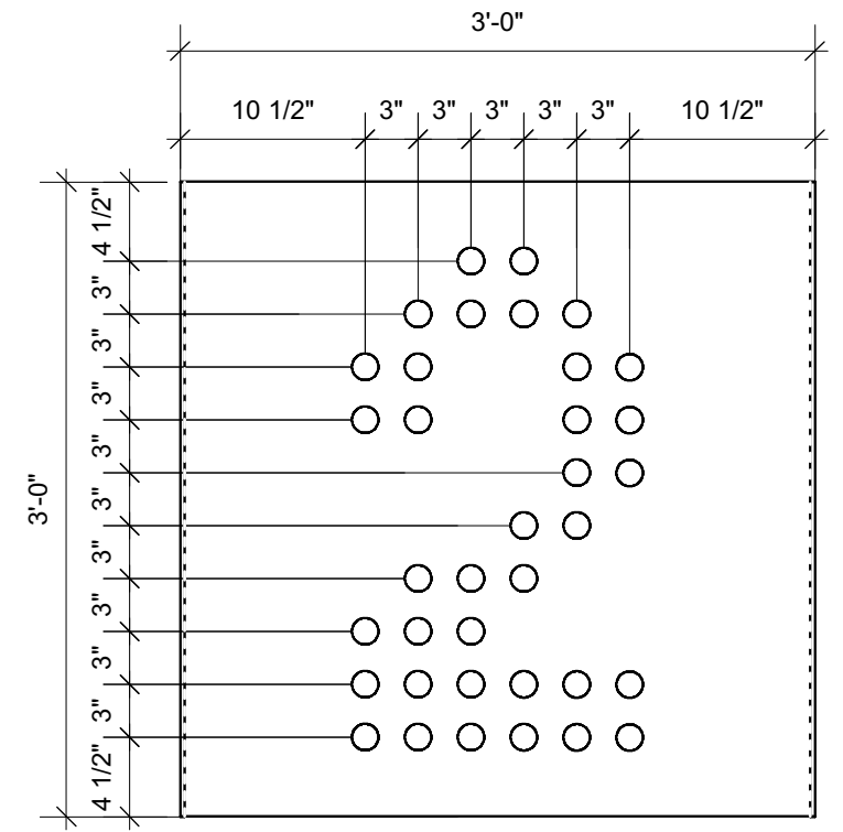
4 Module B05 Scale: 1" = 1'-0"
