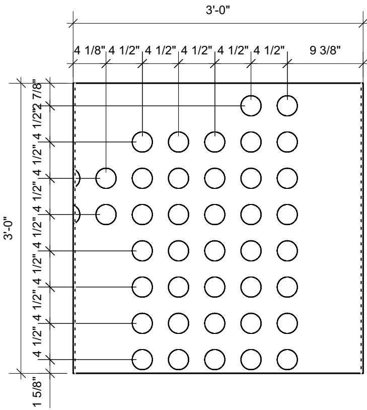
1 Module B02 Scale: 1" = 1'-0"
