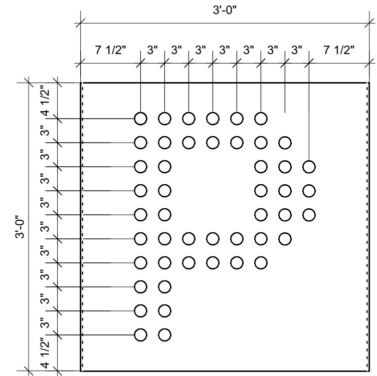
4 Module C06 Scale: 1" = 1'-0"
