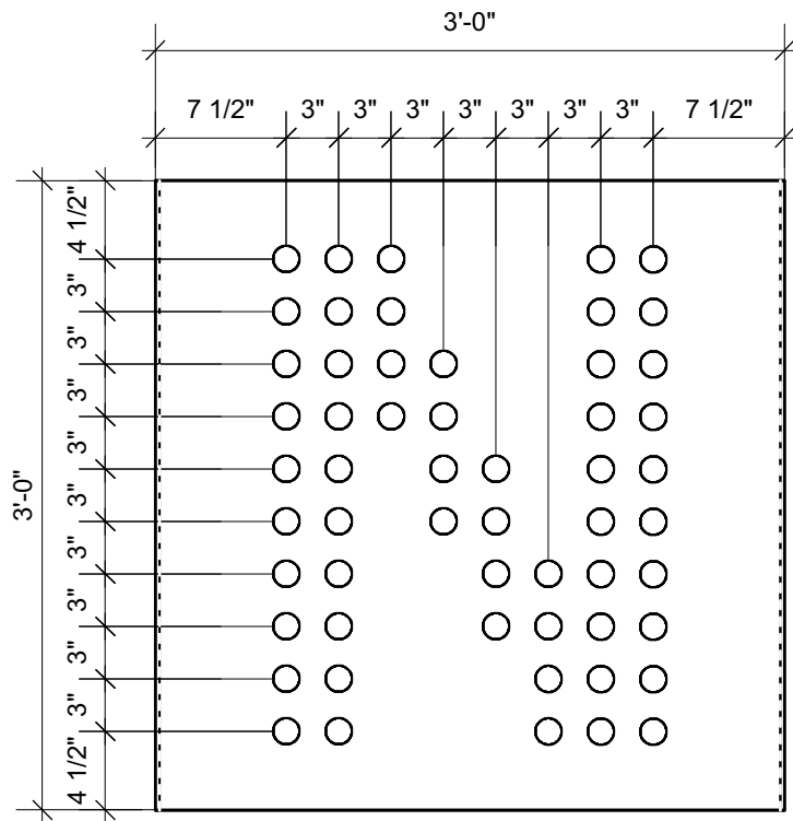
1 Module C03 Scale: 1" = 1'-0"
