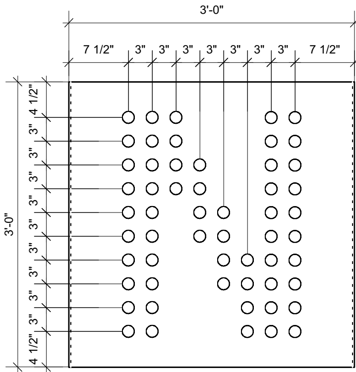
2 Module C04 Scale: 1" = 1'-0"
