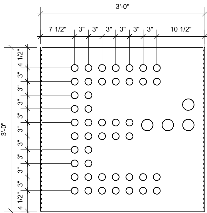
5 Module C07 Scale: 1" = 1'-0"
