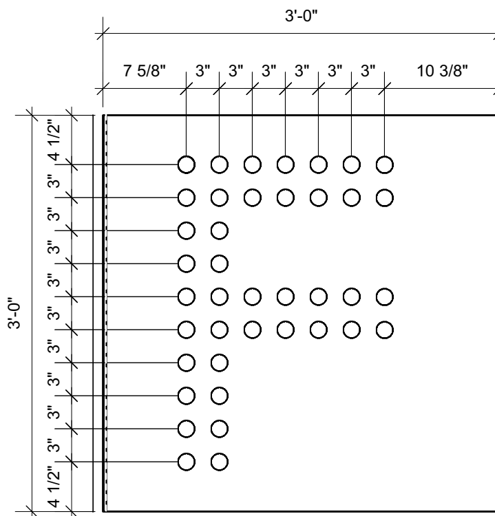
7 Module C09 Scale: 1" = 1'-0"
