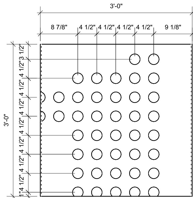
6 Module C08 Scale: 1" = 1'-0"
