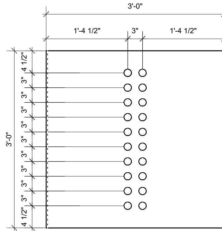
3 Module C05 Scale: 1" = 1'-0"
