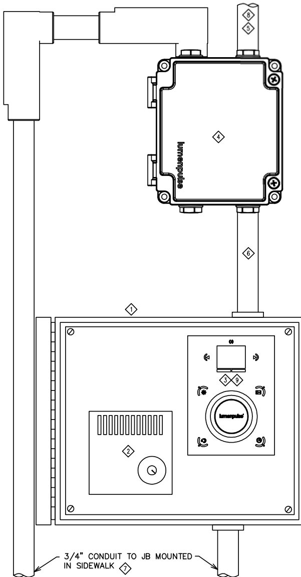
1 DMX CONTROL & ENCLOSURE E4.0 SCALE: N.T.S.
