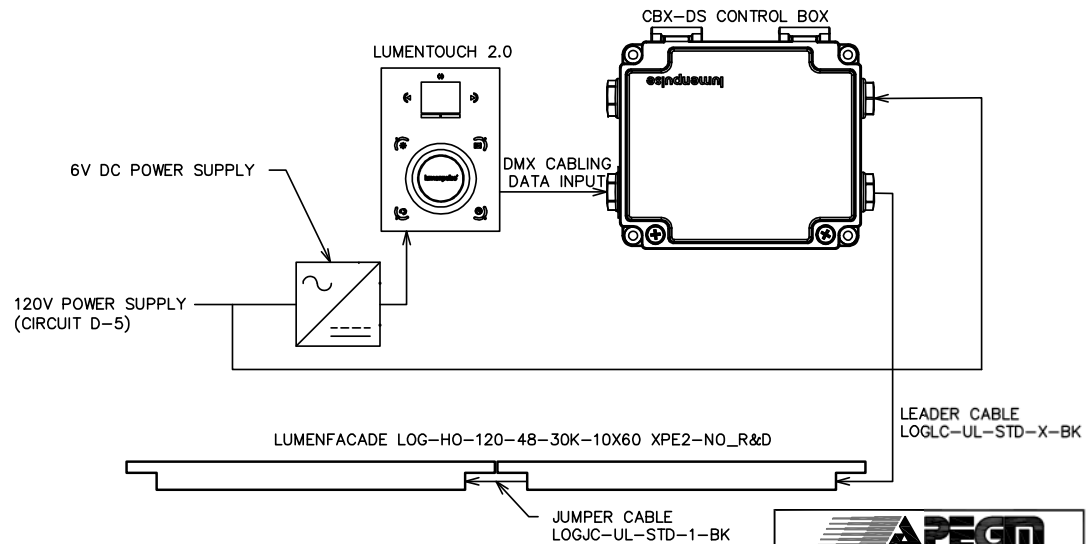
2 DMX CONTROL WIRING SCHEMATIC E4.0 SCALE: N.T.S.
