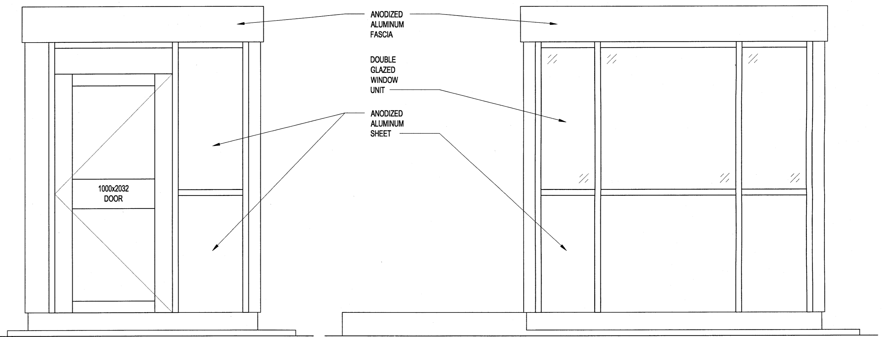
C KIOSK - ELEVATION SCALE: 1:20
