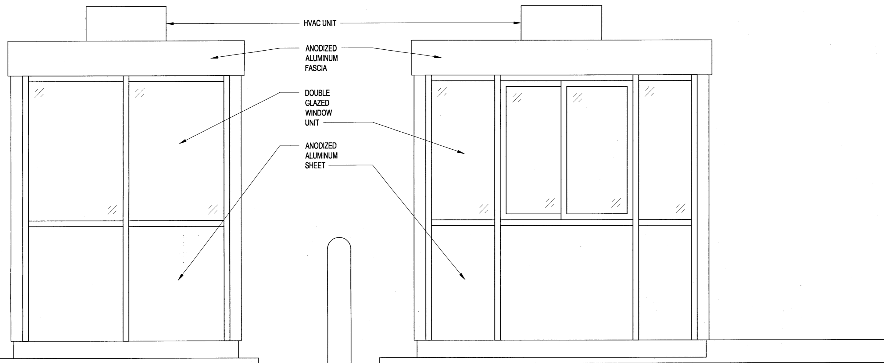
A KIOSK - ELEVATION SCALE: 1:20
